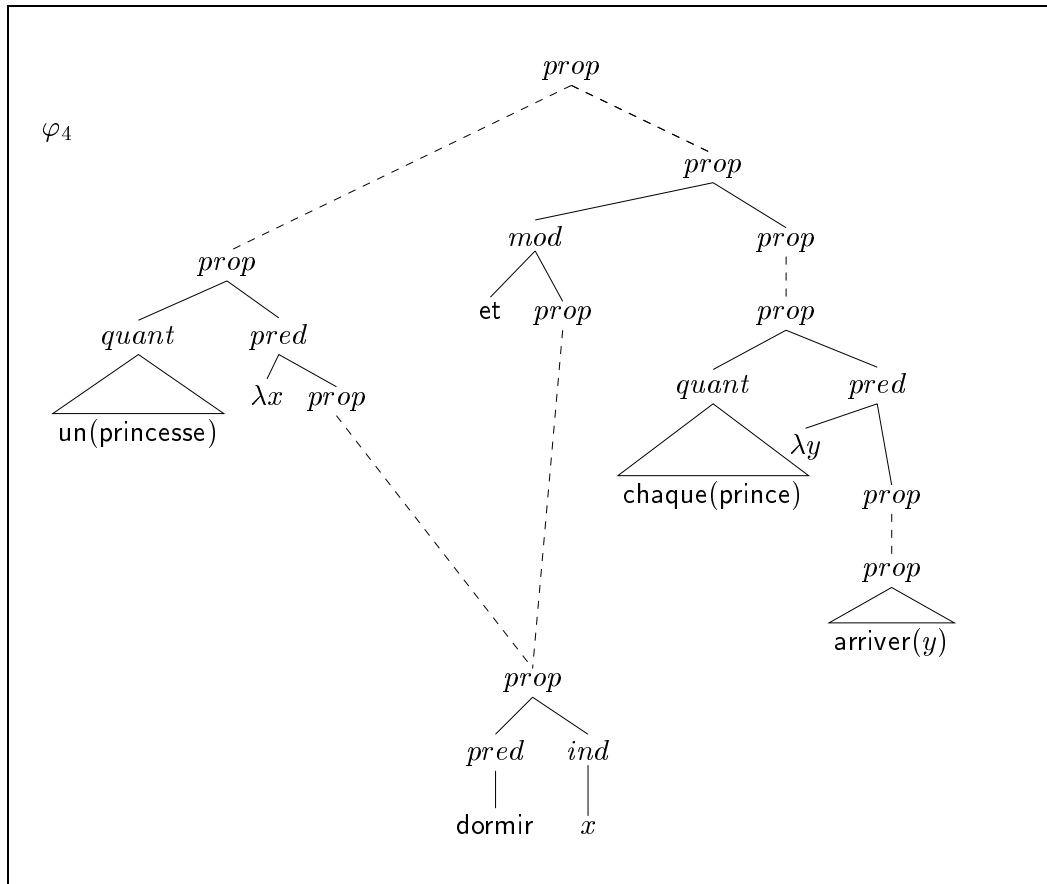
FIGURE 5.32: DESCRIPTION DERIVED IN G_{sem} FOR une princesse dort et chaque prince arrive
