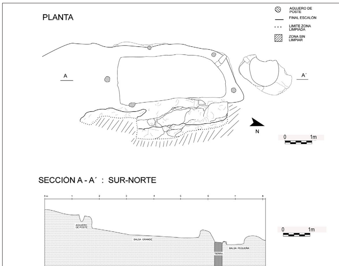
Figura 6. Planta y sección del lagar rupestre de Rincón de Herreros o Pililla del Moro Eusebio.
