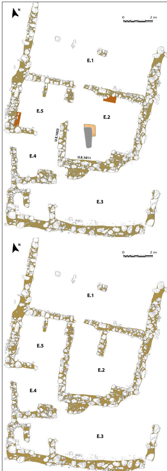
Figura 7. Planta de la bodega de Rambla de la Alcantarilla: Fase 1 (arriba), Fase 2 (abajo).
