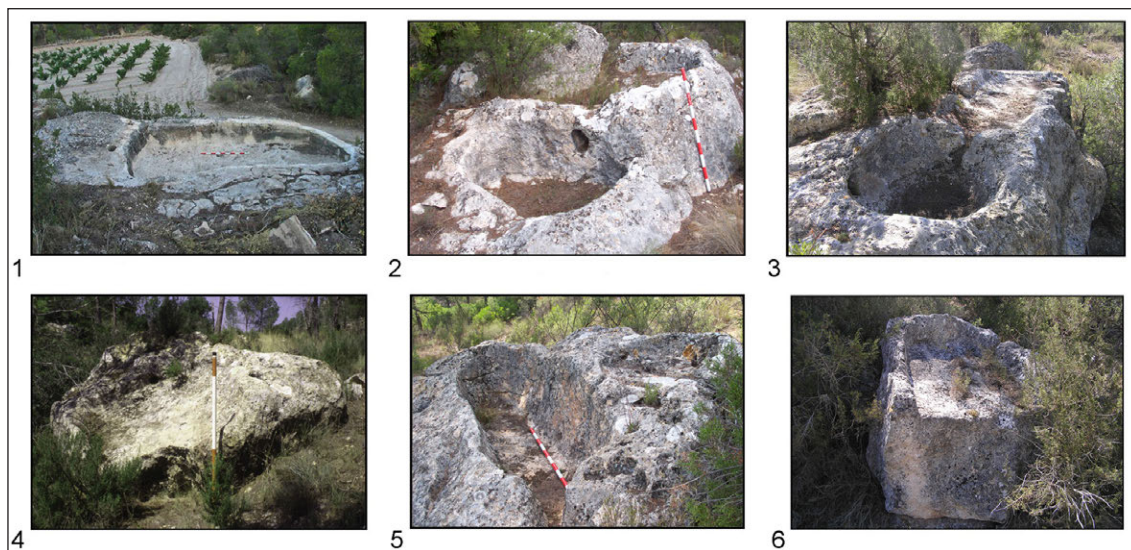
Figura 5. Lagares rupestres: 1, Rincón de Herreros o Pililla del Moro Eusebio; 2, 3 y 4 Rambla de la Alcantarilla; 6, Solana de las Carbonerillas. Almazara rupestre: 5, Solana de Cantos 2.
