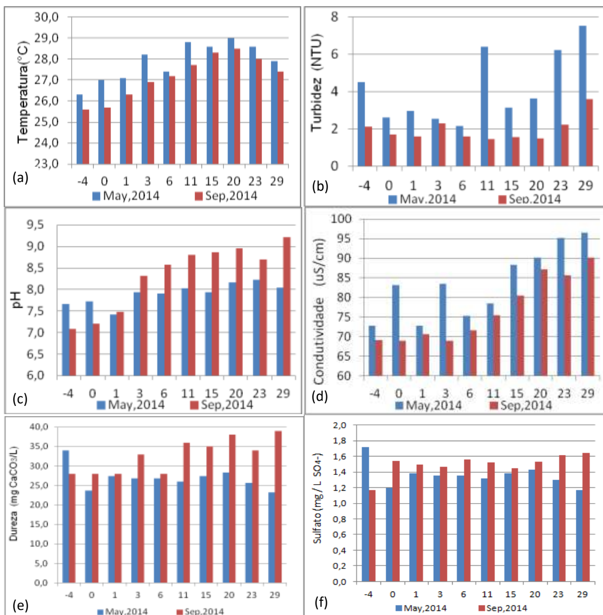
Figura 5 – Evolução das parâmetros de (a) temperatura, (b) turbidez, (c) pH, (d) condutividade, (e) dureza total, (f) sulfato ao longo do Canal do Sertão Alagoano para as duas coletas estudadas (maio e setembro de 2014 ambas em período seco).
