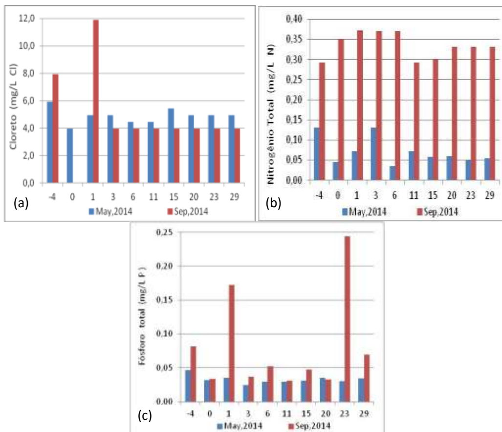
Figura 6 – Evolução dos parâmetros de (a) cloreto, (b) nitrogênio total e (c) fósforo total ao longo do Canal do Sertão Alagoano para as duas coletas estudadas (maio e setembro de 2014 ambas em período seco).
