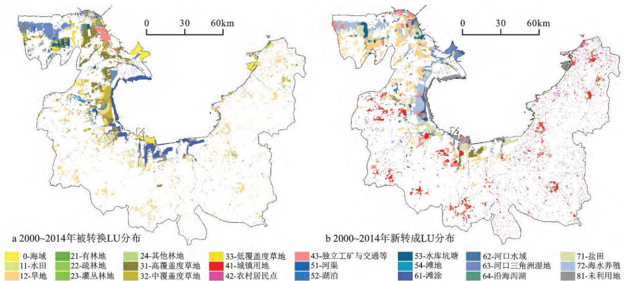
图2 莱州湾土地利用空间格局转移特征分布,2000~2014年 Fig.2 Change of land use/land cover of Laizhou Bay coastal zone in 2000-2014
