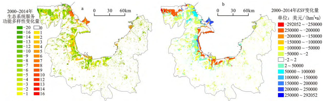
图3 2000~2014年土地利用变化导致的生态系统服务功能多样性变化及价值变化 Fig.3 Change of ecosystem service functions and values caused by land use change in 2000-2014
