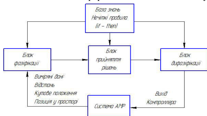
Рис. 1. Структура нечіткого контролера системи
