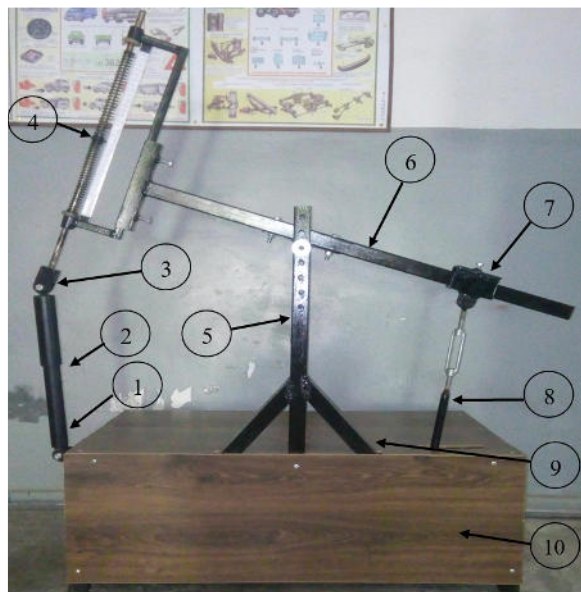
Рис. 1. Стенд для перевірки та визначення робочих параметрів амортизаторів: 1 – нижнє кріплення амортизатора; 2 – амортизатор; 3 – верхнє кріплення амортизатора; 4 – динамометричний механізм; 5 – стійки; 6 – коромисло; 7 – повзун; 8 – шатун; 9 – корпус; 10 – захисна обшивка.
