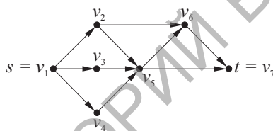
Рис. 1. Орграф H
