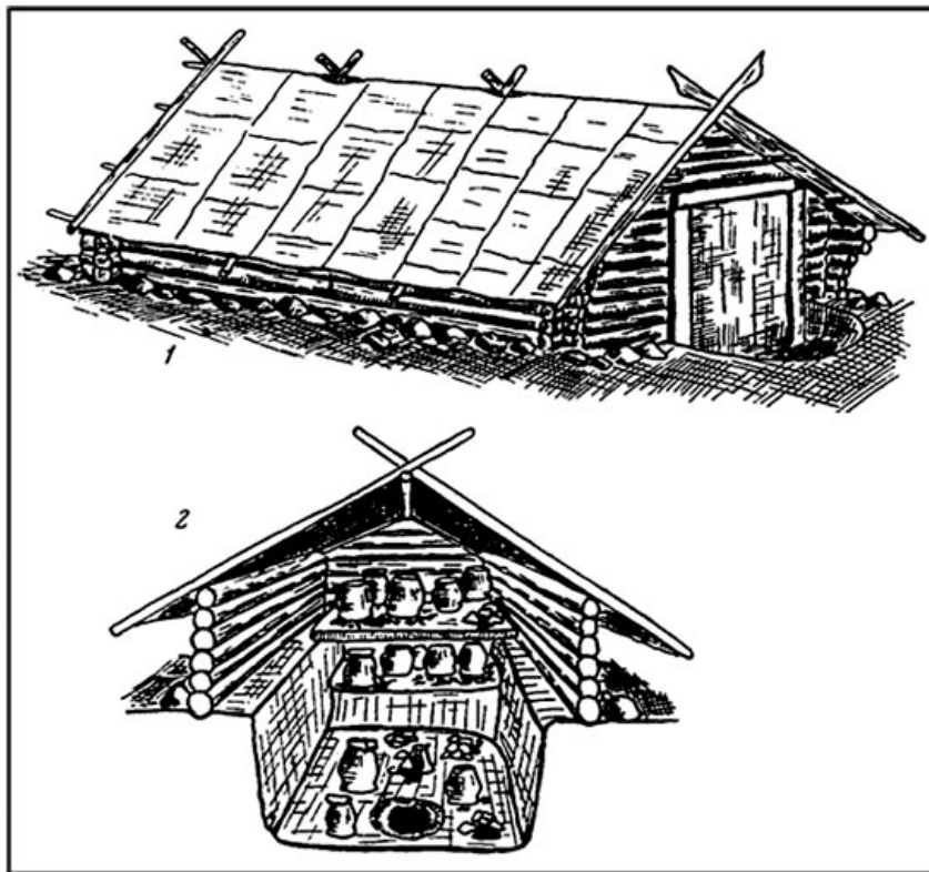
Рис. 5. Опыт реконструкции внешнего (1) и внутреннего (2) вида погребального сооружения на городище близ бывшего Саввино-Сторожевского монастыря (реконструкция авторов раскопок)
