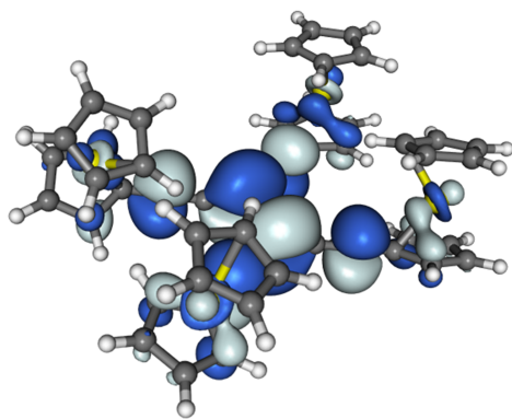
LUMO [1]
