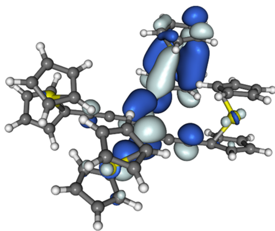
SOMO [1] +
