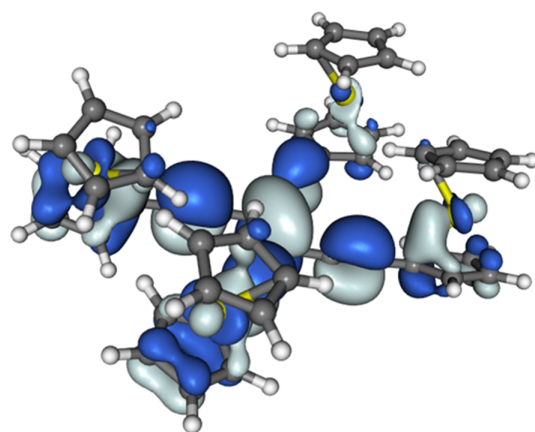
HOMO [1] +
