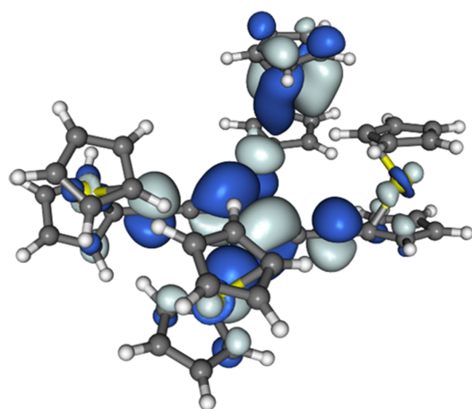
LUMO [1] +
