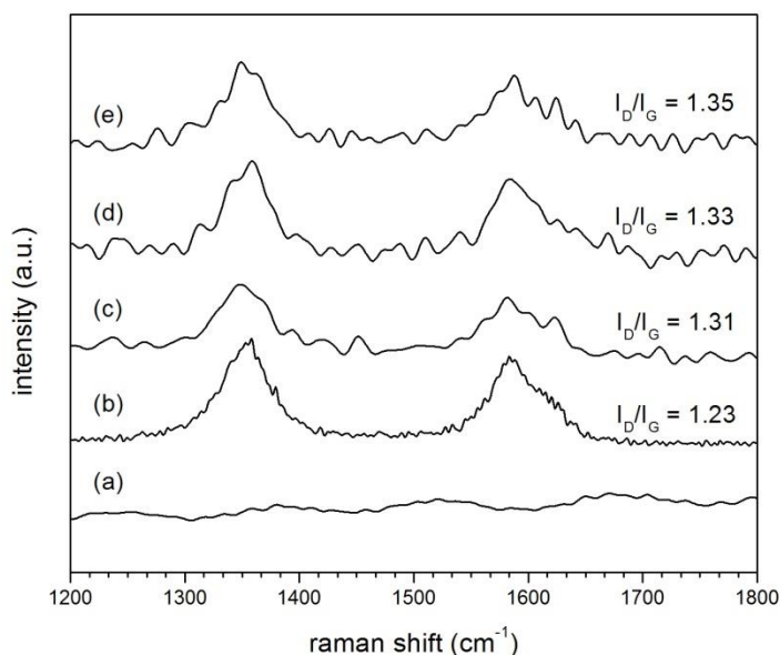
Fig. 6 Raman spectra of (a) NR-latex matrix, (b) MWCNTs, (c) MWCNTs/NR-latex, (d) MWCNTs/NR-latex/SDS, and (e) MWCNTs/NR-latex/TC14.
