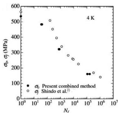
Fig. 2. S-N diagrams at 4 K.
