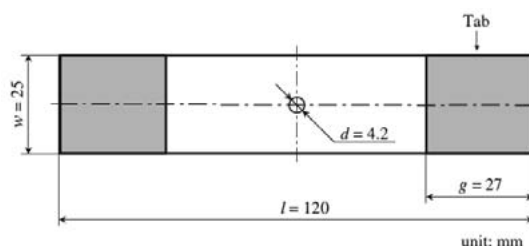
Fig. 1. Open hole specimen.
