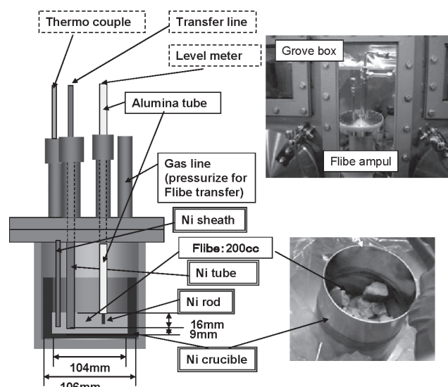
Fig. 2 Flibe ampul
