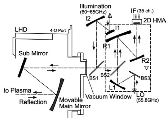
Fig. 1. MIR optics system in LHD.
