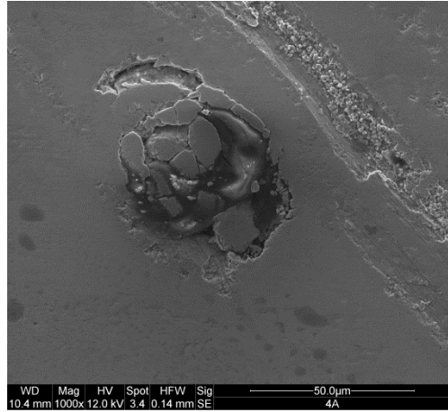
Figure 4.49: DI Gray (50X, 1000X)
