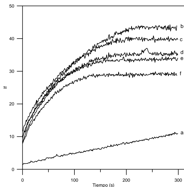
Figura IV.8. Curvas cinéticas de la oxidación de 1 \mu\text{g mL}^{-1} de MTX con \text{KMnO}_4 3.3 \times 10^{-5} M, en función de la concentración de tampón: a) 0 M, b) 0.017 M, c) 0.05 M, d) 0.12 M, e) 0.17 M, f) 0.3 M.
