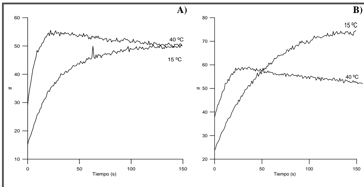
Figura IV.17. Curvas cinéticas registradas a \lambda_{exc/em} = 274/446 \text{ nm} (A) y \lambda_{exc/em} = 247/469 \text{ nm} (B).
