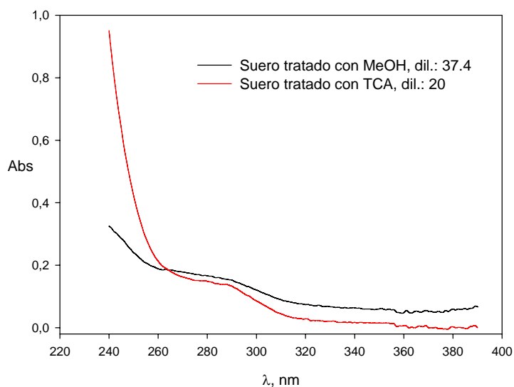
Figura VI.18. Espectros de absorbancia de muestras de suero equino sometidas a procesos de desproteneización con TCA (dilución = 20) y MeOH (dilución = 37).
