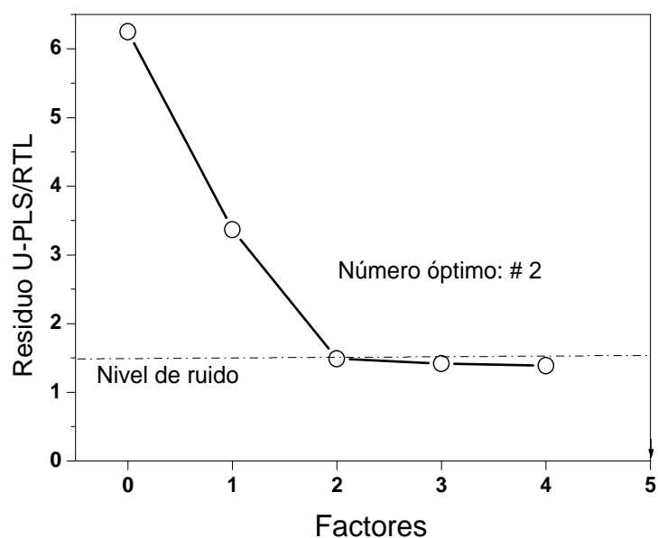
Figura IV.43. Representación de los residuos de predicción ( s_u ) en función del número de interferentes ( N_{int} ) para la muestra de suero 2, que contiene 0.34 \text{ mg mL}^{-1} de AF y 0.34 \text{ mg mL}^{-1} de MTX. El nivel de ruido en este sistema es de 1.5 unidades relativas de fluorescencia (---).
