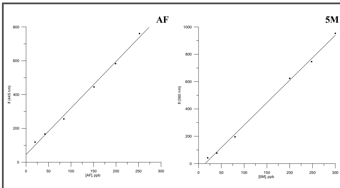
Figura V.21. Influencia de la concentración de AF y 5M en la señal de fluorescencia. pH 4, T = 15 °C, \lambda_{ex} = 275 \text{ nm} .
