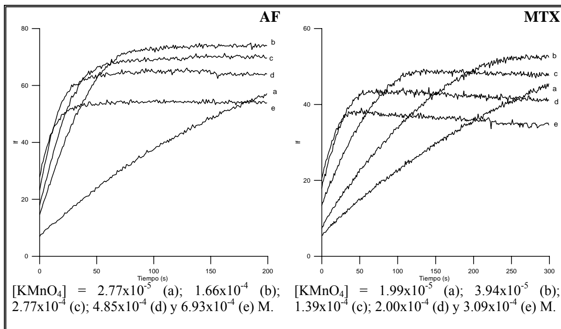
Figura IV.12. Curvas cinéticas de la oxidación de 1 \mu\text{g mL}^{-1} de AF y MTX en función de la concentración de KMnO_4 .
