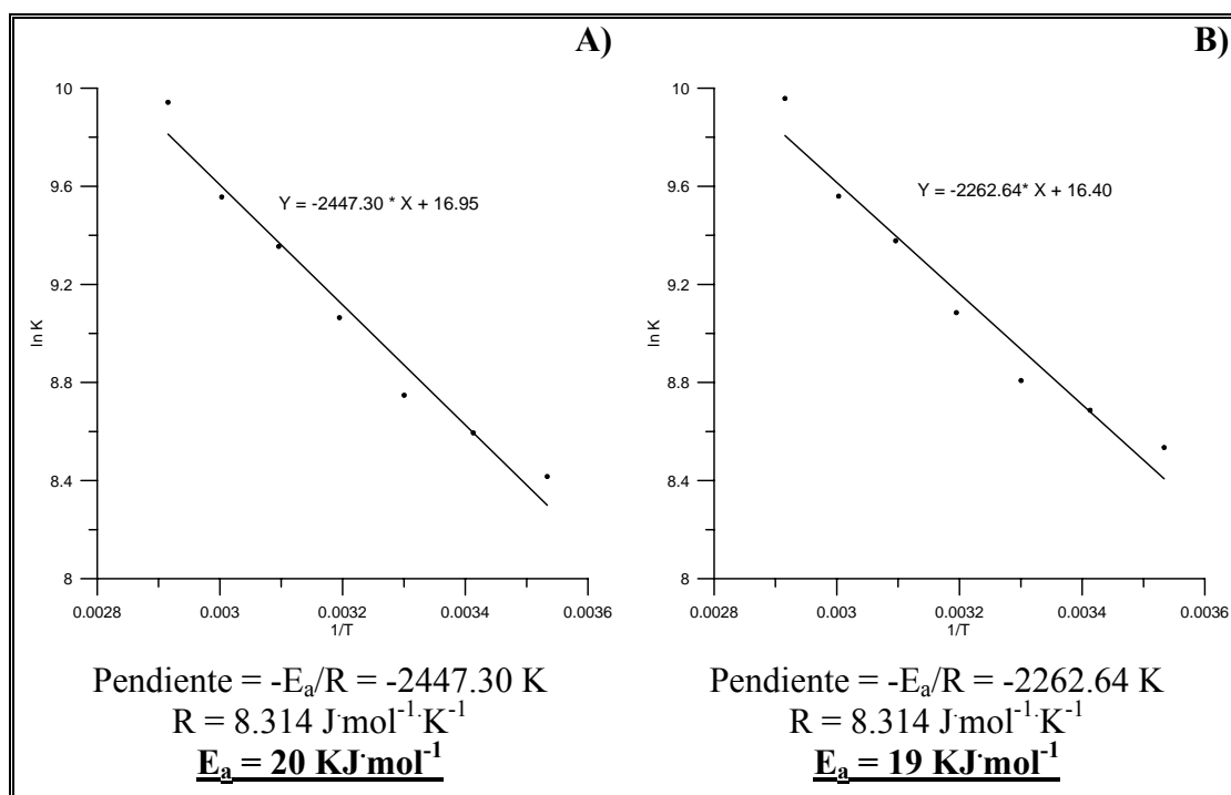
Figura I.25. Cálculo de la energía de activación de la reacción de hidrólisis de quinalfos. [\text{quinalfos}] = 6.7 \times 10^{-6} M. Velocidad determinada entre t_0 : 10 y t_f : 60 seg, A) y velocidad determinada en \Delta t : 50 seg, B).
