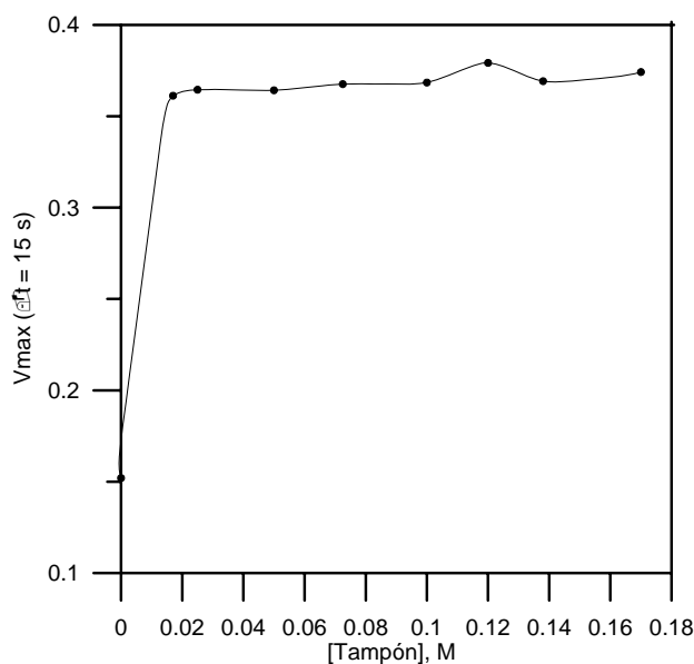
Figura IV.9. Influencia de la concentración de tampón en la oxidación de 1 \mu\text{g mL}^{-1} de MTX con \text{KMnO}_4 3.3 \times 10^{-5} M.
