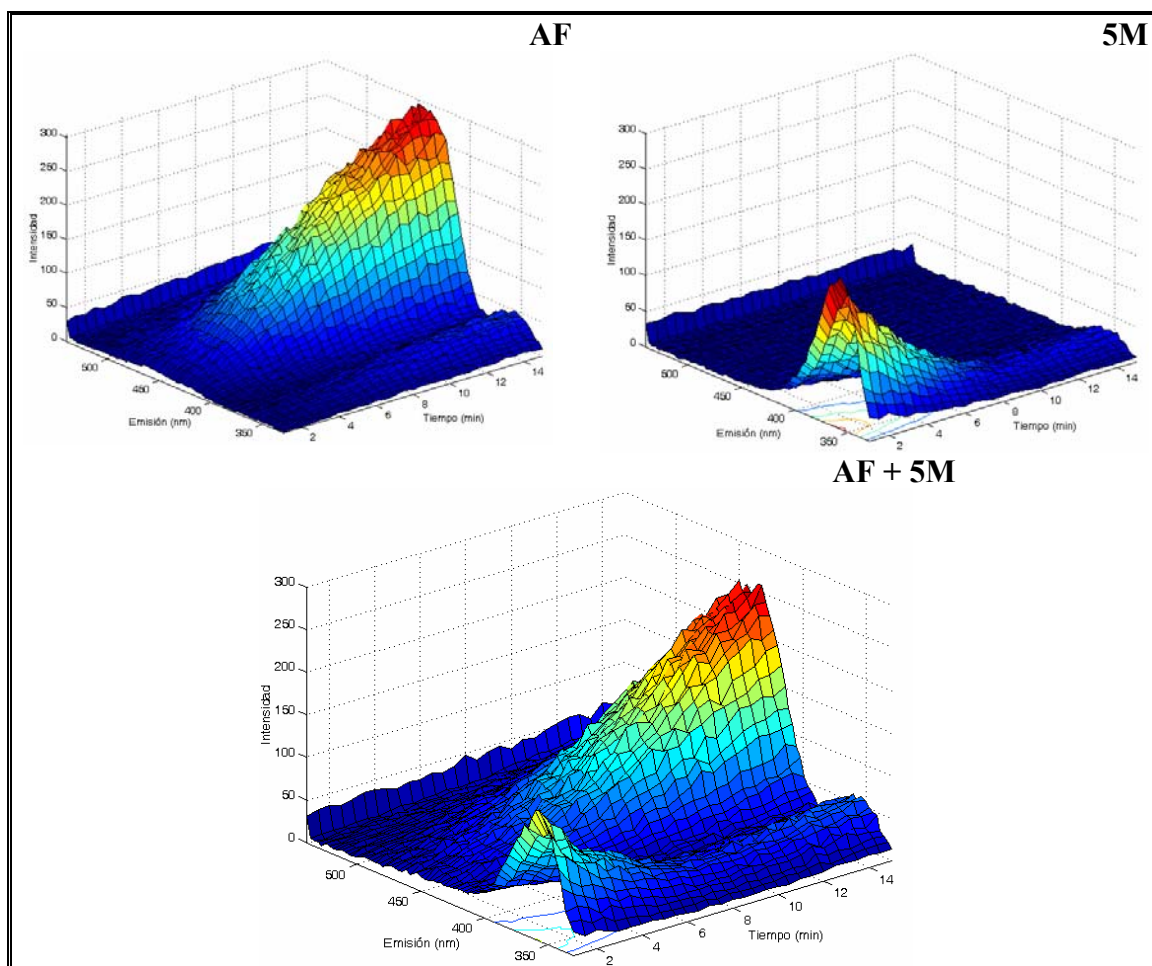
Figura V.22. Evolución de los espectros de emisión de fluorescencia con el tiempo de irradiación de disoluciones de AF, 5M y de una mezcla de ambos analitos.
