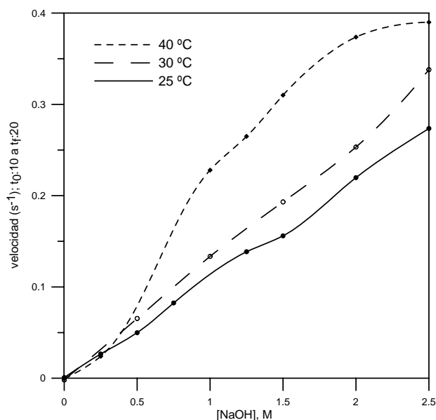
Figura I.32. Variación de la velocidad de reacción de hidrólisis del quinalfos en función de la concentración de NaOH a distintas temperaturas. [quinalfos]: 0.28 \mu\text{g mL}^{-1} .
