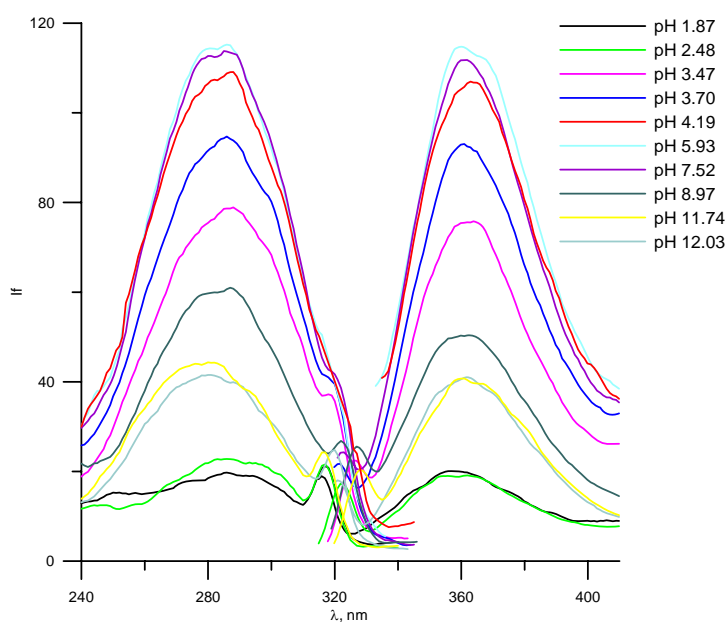
Figura V.6. Espectros de excitación y emisión del ácido THF en función del pH. \lambda_{ex} = 293 \text{ nm} , \lambda_{em} = 362 \text{ nm} ; Voltaje del fotomultiplicador = 700 \text{ V} ; Rendijas ex/em = 5/5 \text{ nm} ; Velocidad de barrido = 10 \text{ nm/seg} ; Temperatura = 20 \text{ }^\circ\text{C} . [\text{THF}] = 0.5 \mu\text{g mL}^{-1}
