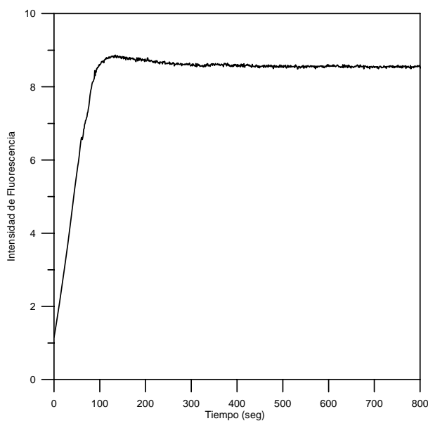
Figura I.9. Curva de hidrólisis de 2 \mu\text{g mL}^{-1} de quinalfos en disolución acuosa al 5 % en etanol, hidróxido sódico 1.5 M. Temperatura = 60 \text{ }^{\circ}\text{C} .
