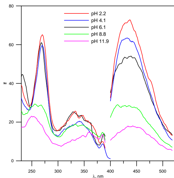
Figura V.5. Espectros de excitación y emisión de AF en función del pH. \lambda_{ex} = 277 \text{ nm} , \lambda_{em} = 445 \text{ nm} ; Voltaje del fotomultiplicador = 800 \text{ V} ; Rendijas ex/em 5/5 \text{ nm} ; Velocidad de barrido = 10 \text{ nm/seg} ; Temperatura = 20 \text{ }^\circ\text{C} . [\text{AF}] = 0.5 \mu\text{g mL}^{-1}
