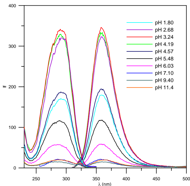
Figura V.7. Espectros de excitación y emisión del ácido 5M en función del pH.: \lambda_{ex} = 290 \text{ nm} , \lambda_{em} = 360 \text{ nm} ; Voltaje del fotomultiplicador = 700 \text{ V} ; Rendijas ex/em = 5/5 \text{ nm} ; Velocidad de barrido = 10 \text{ nm/seg} ; Temperatura = 20 \text{ }^\circ\text{C} . [5M] = 0.5 \mu\text{g mL}^{-1}
