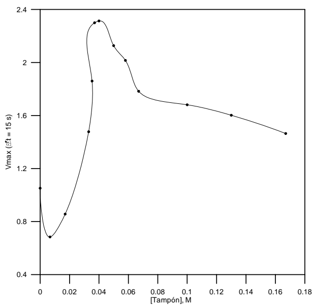
Figura IV.11. Influencia de la concentración de tampón en la cinética de oxidación de 1 \mu\text{g mL}^{-1} de AF con \text{KMnO}_4 3.3 \times 10^{-5} M.
