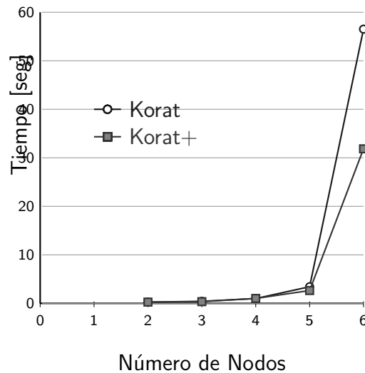
Figura 6.9: Tiempos de corrida de Korat y Korat+ para Árboles binarios de búsqueda ( search )
