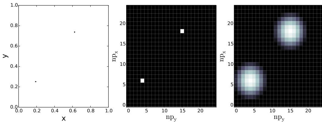
Fig. A.2 Ejemplo de la representación de una campo de densidad subyacente trazado por dos partículas puntuales. El panel izquierdo muestra un gráfico típico de las partículas en una dada proyección. El panel del medio muestra la imagen resultante luego de dividir el espacio en 25x25 píxeles cuadrados. El panel derecho muestra la imagen resultante luego de esparcir la masa de las partículas adentro de un dominio de influencia dado.
