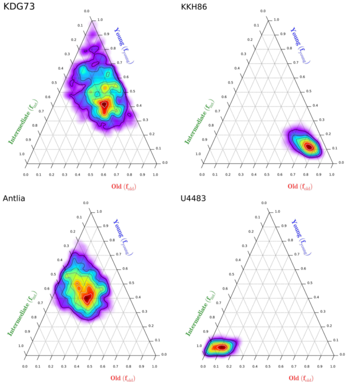
Fig. 3.10 Ejemplos de diagramas ternarios que resumen las historias de formación estelar de las galaxias enanas KDG73, KKH86, Antlia y U4483. Los colores indican la distribución de probabilidades de f_{old} , f_{int} , y f_{young} luego de tener en cuenta las incertezas del modelo. (Ver la barra de color en la Figura 3.11.)
