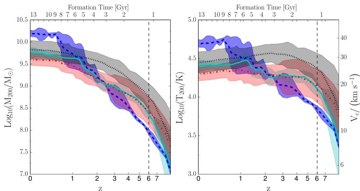
Fig. 3.7 Evolución de la masa virial, M_{200} , (panel izquierdo) y de la temperatura virial, T_{200} , (panel derecho) de los progenitores principales de las galaxias enanas simuladas, separadas en cuatro grupos según sus historias de formación estelar identificadas en la Figura 3.5. Las distintas líneas indican el promedio para cada grupo; Las áreas sombreadas indican la dispersión para cada tiempo. Note que la pertenencia a cada grupo está determinada por la masa (o temperatura virial) del progenitor en z_{\text{reion}} . Aquellos sistemas más masivos en z_{\text{reion}} (línea gris punteada) inician la formación estelar antes de la reionización y la sostienen durante varios Gyr . Los sistemas menos masivos en z_{\text{reion}} son más susceptibles a la reionización cósmica, la cual induce un decrecimiento pronunciado en la actividad de formación estelar en tiempos intermedios ( f_{\text{int}} < 0.2 ). De todas las galaxias del último grupo, las menos masivas en z_{\text{reion}} forman estrellas principalmente en tiempos tardíos (línea a trazos azul), mientras que las más masivas experimentan un único episodio de formación estelar temprano (línea a trazos punteada). Los sistemas con dos componentes estelares de distinta edad (línea sólida cian) resultan de una fusión tardía que dispara un evento de formación estelar reciente en un sistema “rojo”.
