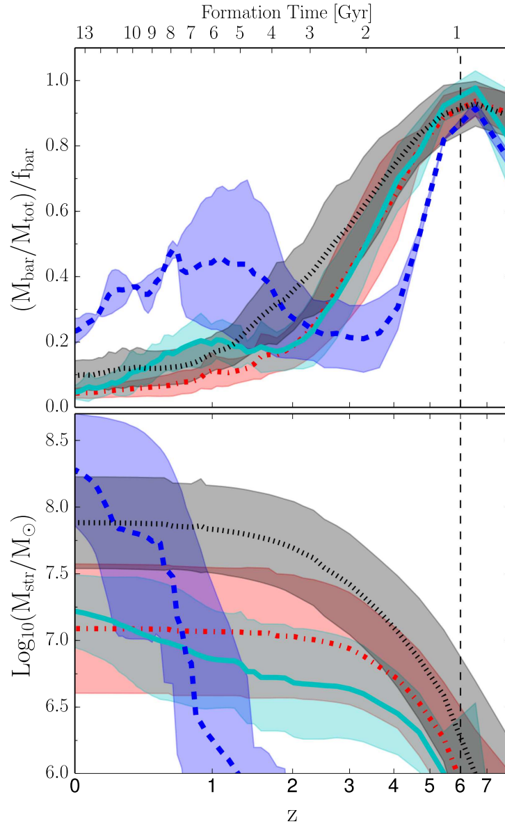
Fig. 3.8 Evolución de la fracción bariónica adentro del radio virial (panel superior) y de la masa estelar (panel inferior) para cada uno de los cuatro grupos identificados en la Figura 3.5 de acuerdo a sus historias de formación estelar. Todas estas galaxias pierden la mayoría de sus bariones debido al efecto de la reionización cósmica y al feedback estelar. La pertenencia a cada grupo refleja la masa del progenitor en z_{\text{reion}} (marcado por una línea vertical a trazos), lo cual determina qué tan rápido pueden ser evacuados los bariones del halo de cada galaxia enana. Los halos mostrados en azul corresponden al progenitor menos masivo en z_{\text{reion}} . Estos sistemas no son lo suficientemente masivos como para comenzar a formar estrellas antes de la reionización, y son, por lo tanto, los halos más severamente afectados cuando el gas es calentado repentinamente en z_{\text{reion}} . El calentamiento empuja al gas hacia afuera del halo e induce un retraso en la formación estelar de estos sistemas. Los sistemas mostrados en rojo son suficientemente masivos como para comenzar a formar estrellas antes de la reionización, pero no lo suficientemente masivos como para retener el gas una vez que la reionización y el feedback comienzan a actuar. Los sistemas mostrados en gris son lo suficientemente masivos como para permitir que una gran cantidad de gas se enfríe y se condense antes de la reionización, lo que permite sostener la formación estelar durante un periodo de tiempo mucho más prolongado. Ver texto para más detalles.
