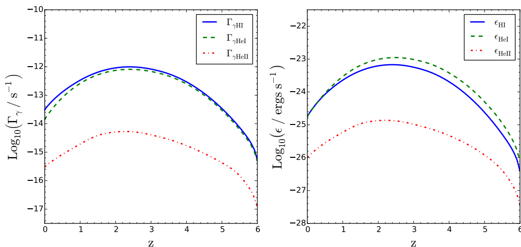
Fig. 1.1 Tasas de fotoionización (panel izquierdo) y foto-calentamiento (panel derecho) para el hidrógeno y el helio como función del redshift . Los cálculos fueron hechos asumiendo el espectro de Haardt and Madau (1996)
