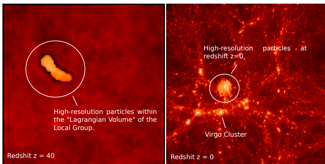
Fig. 1.2 Distribución de materia oscura adentro de una caja de \sim 87.7 Mpc en redshift z = 40 (panel izquierdo) y redshift z = 0 (panel derecho). Esta figura muestra cómo se lleva a cabo la técnica de zoom-in para incrementar la resolución de la región en la cuál se forma el Grupo Local. El volumen lagrangiano del Grupo Local es llenado por un gran número de partículas de baja masa. Las partículas afuera de este volumen aseguran que los efectos tidales debido a las estructuras en gran escala, tales el cúmulo de Virgo, operen sobre el Grupo Local. Las imágenes fueron renderizadas con el código de visualización Py-SPHViewer (ver el apéndice A para detalles).
