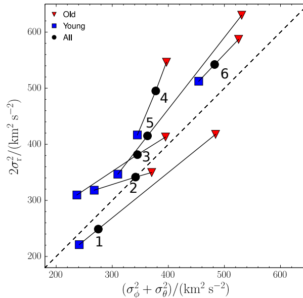
Fig. 4.3 Correlación entre la dispersión de velocidad radial y transversal para las seis galaxias enanas con “dos componentes”. Los círculos negros corresponden al total de la galaxias, mientras que los cuadrados azules y los triángulos rojos corresponden a la población joven y vieja respectivamente. La línea a trazos muestra la relación esperada en ausencia de anisotropía orbital. Las líneas negras sólidas conectan los valores obtenidos para todas las estrellas, la población joven y la población vieja. Es interesante notar que la población joven es más dinámicamente fría que su contraparte vieja. A pesar de que no lo mostramos aquí, el mismo comportamiento se observa cuando se divide el contenido estelar de acuerdo a la metalicidad.
