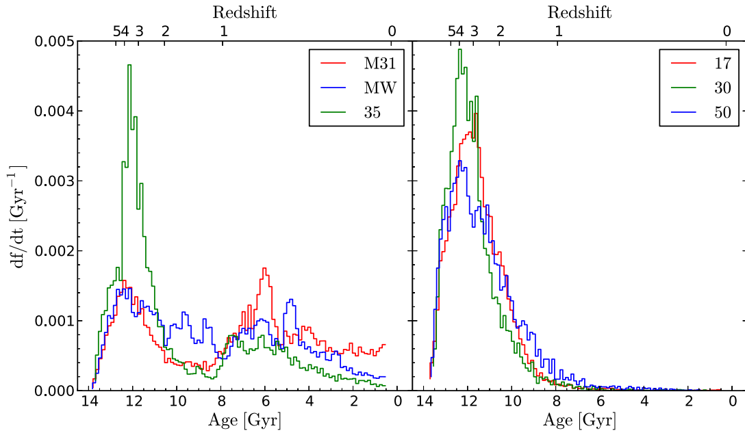
Fig. 2.3 Historia de formación estelar de las galaxias despojadas de sus envoltentes gaseosas debido a su interacción con la “telaraña” o “red” cósmica (panel derecho). Los histogramas muestran la distribución de las edades estelares de tres galaxias cuyas trayectorias se trazan en la Figura 2.1. Todos estos sistemas atraviesan un “panqueque” de gran escala aproximadamente al mismo tiempo, z \sim 2 , y este es el momento cuando ellas son despojadas de la mayor parte de su gas. Sin este reservorio de gas, la formación estelar cesa poco tiempo después, una vez que el gas restante y denso es transformado en estrellas. Por el contrario, la formación estelar en halos que no son afectados por este mecanismo puede continuar hasta el presente. Estas son galaxias que no cruzan ningún filamento durante su evolución, o que son lo suficientemente masivas para resistir la interacción. En el panel izquierdo mostramos tres ejemplos.
