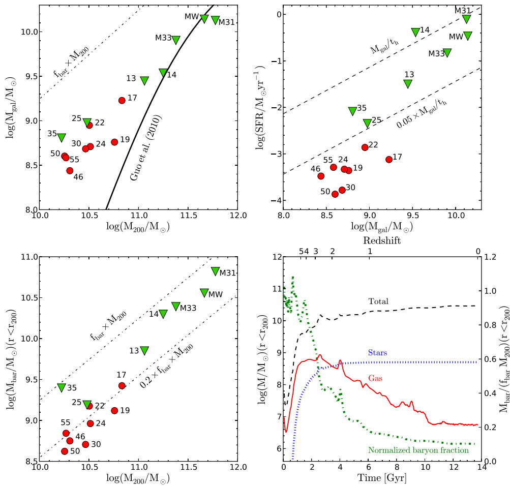
Fig. 2.2 Masa estelar adentro del radio galáctico (panel superior izquierdo) y masa bariónica total adentro del radio virial (panel inferior izquierdo) en función de la masa virial del halo. El panel superior derecho muestra la tasa de formación estelar actual en función de la masa estelar de las galaxias. Pueden identificarse dos poblaciones: (i) galaxias que forman estrellas con tasas comparables a su tasa de formación estelar promedio (triángulos verdes), y (ii) aquellas en donde la formación estelar ha cesado (triángulos rojos). Las galaxias de este último grupo han perdido más del \sim 80\% de sus bariones disponibles. A una dada masa de halo, estas galaxias han formado sustancialmente menos estrellas que sus contrapartes formadoras, lo que sugiere que la pérdida de bariones y la falta de formación estelar no se debe al feedback estelar. La evolución de la masa adentro del radio virial de una de estas galaxias (galaxia “30”) ilustra la pérdida repentina de bariones que resulta del efecto de la “presión de barrido” luego de cruzar un “panqueque” de la estructura en gran escala a z \sim 2 (panel inferior derecho). La masa virial es prácticamente el doble luego de esto, pero la masa total bariónica apenas crece; en z = 0 el contenido bariónico del halo es menos del 10% de lo esperado de la fracción universal.
