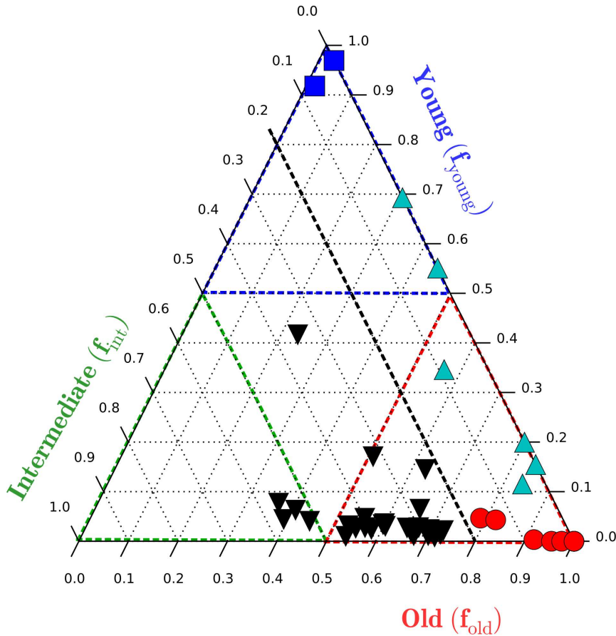
Fig. 3.5 Igual que la Figura 3.2 pero para la muestra de galaxias simuladas. Las poblaciones estelares “joven”, “intermedia”, y “vieja” se refieren aquí a los tiempos de formación encerrados entre t = 3 y 6 \text{ Gyr} . Los sistemas a la derecha de la línea negra a trazos son aquellos con un “hueco” de estrellas de edad intermedia, es decir, f_{int} < 0.2 . De todos ellos, hemos identificado sólo aquellos en los cuales está presente una única poblaciones estelar “vieja” (círculos rojos, f_{young} < 0.1 ); aquellos en donde domina una única población “joven” (cuadrados azules, f_{old} < 0.1 ); y aquellos con dos poblaciones estelares con edades distintas (triángulos cían). Los triángulos negros que apuntan hacia abajo denotan sistemas con f_{int} > 0.2 .
