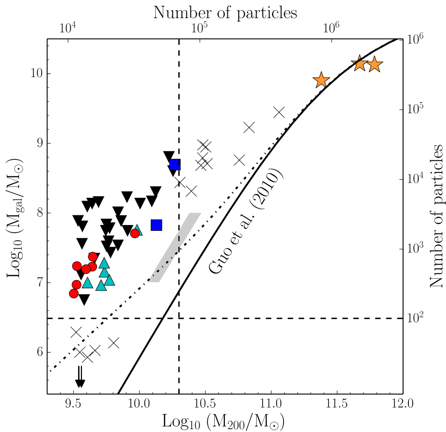
Fig. 3.1 Masa estelar vs masa virial de galaxias centrales en el volumen de la simulación CLUES en z = 0 . Hemos retenido para nuestro análisis a todas las galaxias enanas en halos resueltos con más de \sim 10^4 partículas ( M_{200} > 3 \times 10^9 M_{\odot} ) pero menos masivos que 2 \times 10^{10} M_{\odot} (línea vertical punteada), ya que es poco probable que halos más masivos sean afectados por la reionización. Algunos de los halos en este rango de masas (7 de 53, mostrados con cruces y flechas negras) tienen M_{\text{gal}} < 3 \times 10^6 M_{\odot} (línea punteada horizontal), y no son considerados en nuestro análisis ya que no podemos medir sus historias de formación estelar con precisión. La línea sólida muestra la relación entre la masa de los halos y la masa de las galaxias a partir de determinaciones a través de la técnica de ajuste de abundancias por Guo et al. (2010); la línea punteada indica la corrección para galaxias débiles sugerida por Sawala et al. (2011); y el área sombreada indica restricciones recientes derivadas por Brook et al. (2014). Los diferentes símbolos y colores identifican distintos grupos de galaxias enanas de nuestra muestra, de acuerdo a sus historias de formación estelar; ver la discusión de la Figura 3.5 para detalles. Las estrellas amarillas indican la posición de las galaxias análogas a la Vía Láctea, M31 y M33 en el volumen simulado; es decir, las tres galaxias más masivas en el volumen simulado.
