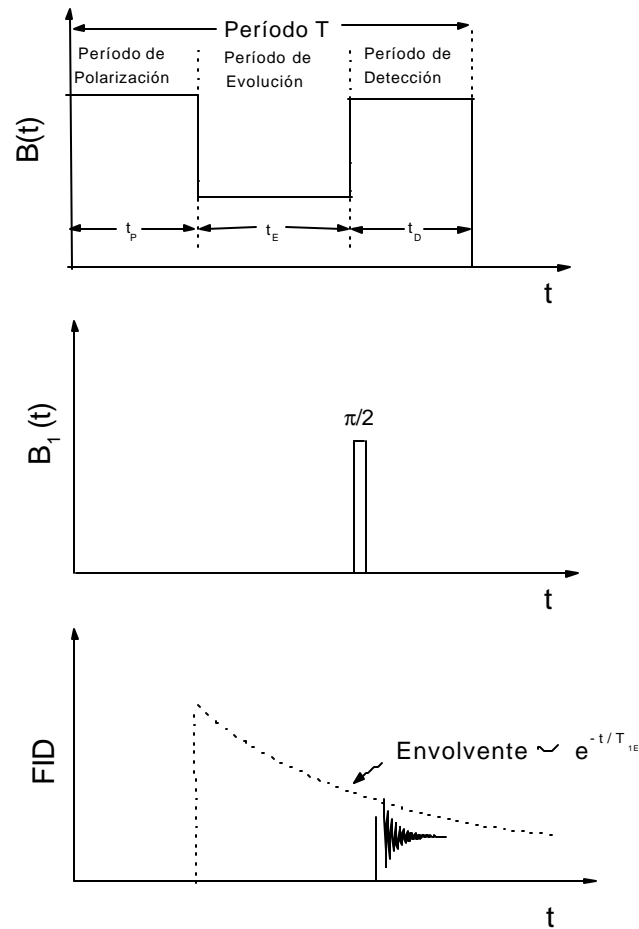
Figura 3.1: En la figura superior se muestra el ciclaje de campo magnético para una medición de T_1 destacándose los períodos involucrados. La figura del centro esquematiza el momento en que se aplica el pulso de radiofrecuencia de \pi/2 . La figura inferior esquematiza la detección de la FID y la medición directa de T_{1E} mediante la construcción de la envolvente.
