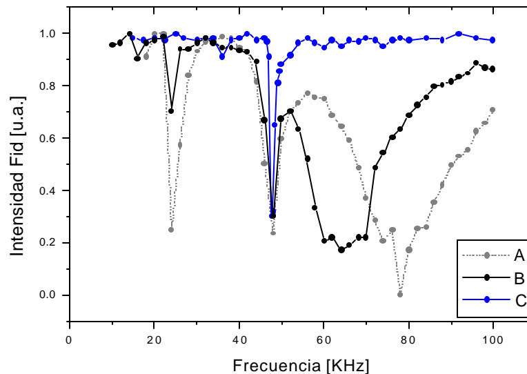
Figura 6.6: Intensidad de la señal de inducción libre para distintos valores de intensidad en la irradiación como función de la frecuencia, con una duración de 100ms. El campo magnético generado por el imán es el correspondiente a una frecuencia de Larmor de 47 KHz. Los amplitud de la señal aplicada corresponde a: A) 8 Vpp, B) 4Vpp y C) 100 mVpp
