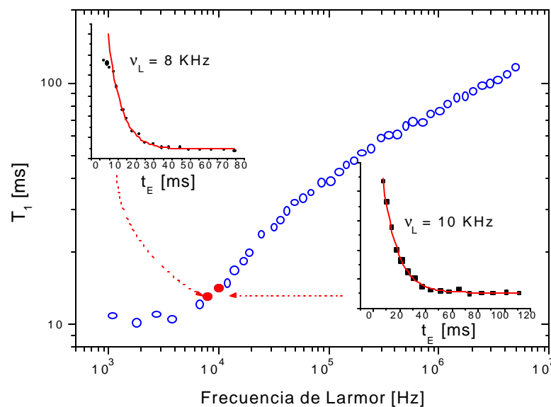
Figura 3.12: Medición del 5CB a 30 0 C en función de la frecuencia de Larmor. Los insertos muestran que por debajo de 10KHz los campos locales influyen en la evolución de la magnetización.
