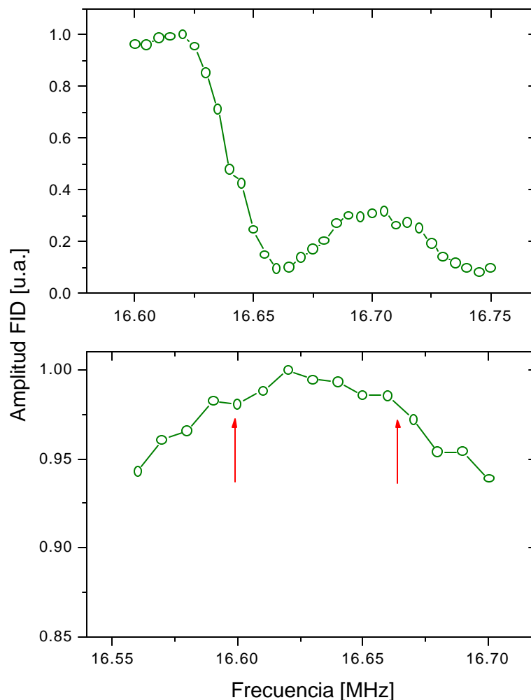
Figura 6.4: Espectro de irradiación del pulso de \pi/2 . En este experimento se mantuvo el campo constante mientras se variaba la frecuencia de irradiación y la de detección, de manera de tener siempre un batido de 20 KHz
