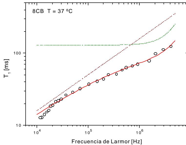
Figura 3.16: Medición del 8CB a 37^{\circ}\text{C} en función de la frecuencia de Larmor en el rango de frecuencias en que se satisface la condición de adiabaticidad. La línea sólida corresponde al ajuste utilizando la ec. (2.12) en donde se ha eliminado el término correspondiente a la frecuencia de corte, y a una rotación alrededor del eje de la molécula, ec. (2.15) con \tau_R = 1.2 \times 10^{-7} seg.
