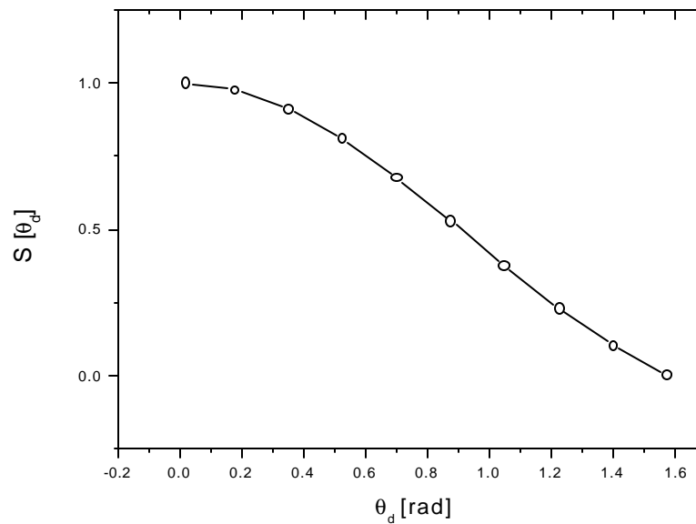
Figura 2.9: Simulación del Parámetro de orden mesoscópico en función del ángulo que forman los directores de los dominios esmécticos respecto del campo magnético externo. Se utilizó una distribución F(\theta_d) = \Theta(\theta_d - \theta_d^m) en (2.5).
