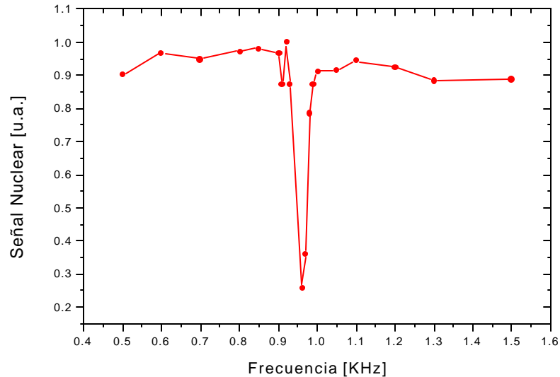
Figura 6.7: Intensidad de la señal nuclear para un experimento de doble resonancia cuando la corriente en el imán es cero. El mínimo corresponde a la frecuencia de precesión de los protones en el campo magnético terrestre.
