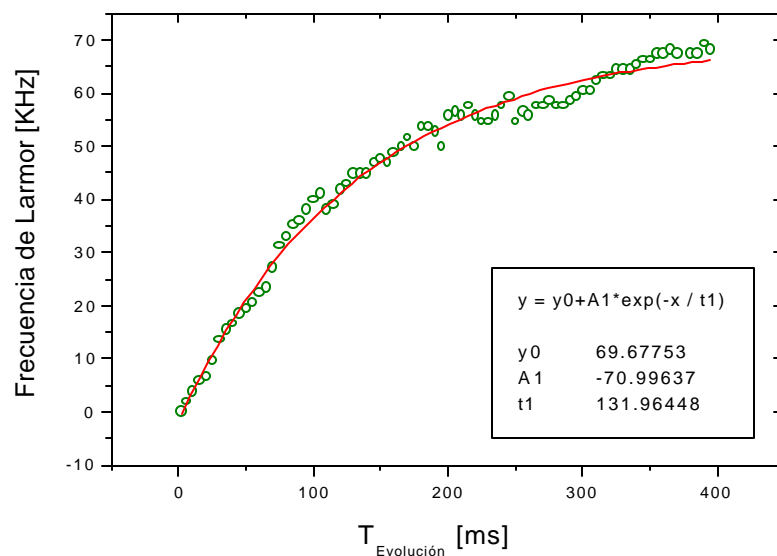
Figura 6.3: Frecuencia de Larmor en función del tiempo de evolución para un tiempo de polarización de 250ms.
