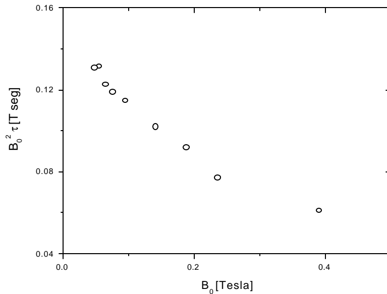
Figura 5.11: B_0^2 \tau vs. B_0 , se observa que el producto no arroja una constante como predice el modelo propuesto.
