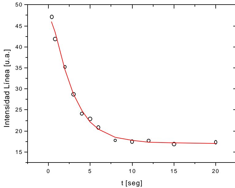
Figura 5.6: Los datos muestran la intensidad de la línea de RMN para un proceso de ordenamiento a 8MHz. La línea sólida corresponde a un ajuste por cuadrados mínimos de (5.9) donde la dependencia temporal de \theta_{max} está dada por la simulación de (5.6) con \theta_0 = \pi/2 .
