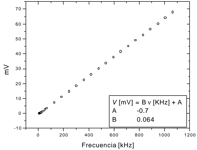
Figura 6.10: Calibración de la escala de 100mV del osciloscopio Nicolet.
