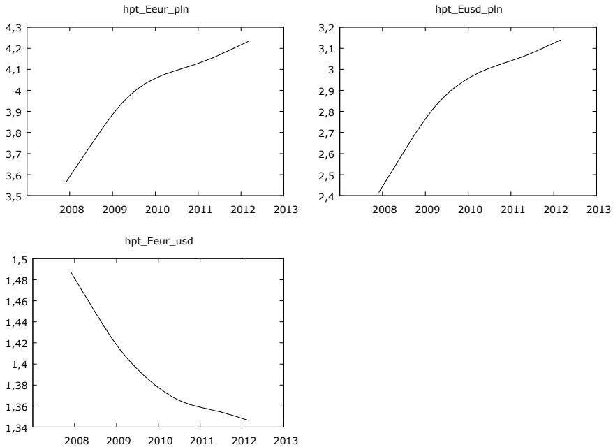
Rysunek 3. Kursy EUR/PLN, USD/PLN i EUR/USD wygładzone przy pomocy filtra Hodricka-Prescotta przy \lambda=14400 w latach 2008–2012
