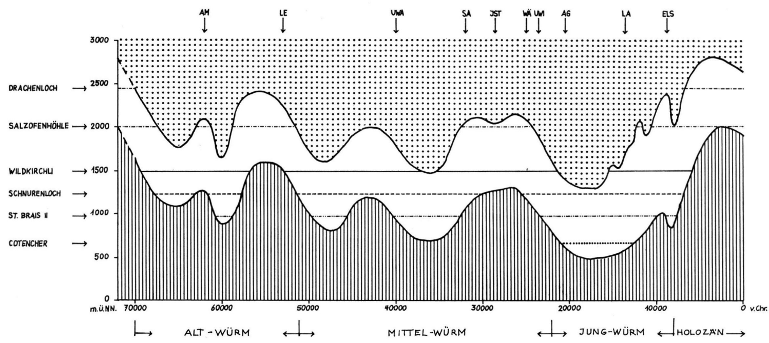
Abb. 1. Schneegrenze und Waldgrenze während der Würm-Eiszeit im nördlichen Alpenbereich. ∴ = ewiger Schnee; ||| = Wald. Am oberen Rand sind einige C 14 -Datierungen angegeben. Die Zeichen bedeuten:
