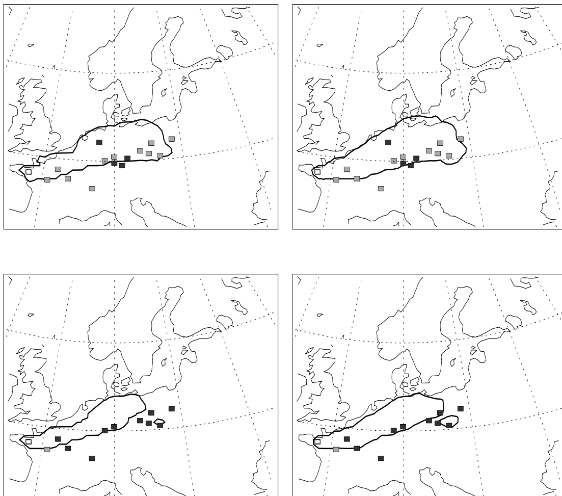
Abbildung 4.5: Die Abbildung zeigt das Ergebnis der Berechnung der pmcp-Ausbreitung. Mit Konturlinien wurde die Verteilung der Partialdichte von 10^{-12} kg/m 3 (oben) und 10^{-11} kg/m 3 (unten) dargestellt. Links sind erneut die mit dem Flußverfahren erzielten Ergebnisse, rechts die nicht-interpolierend berechneten Resultate. Die Markierung mit Symbolen entspricht den Angaben der Tabelle 4.2.
