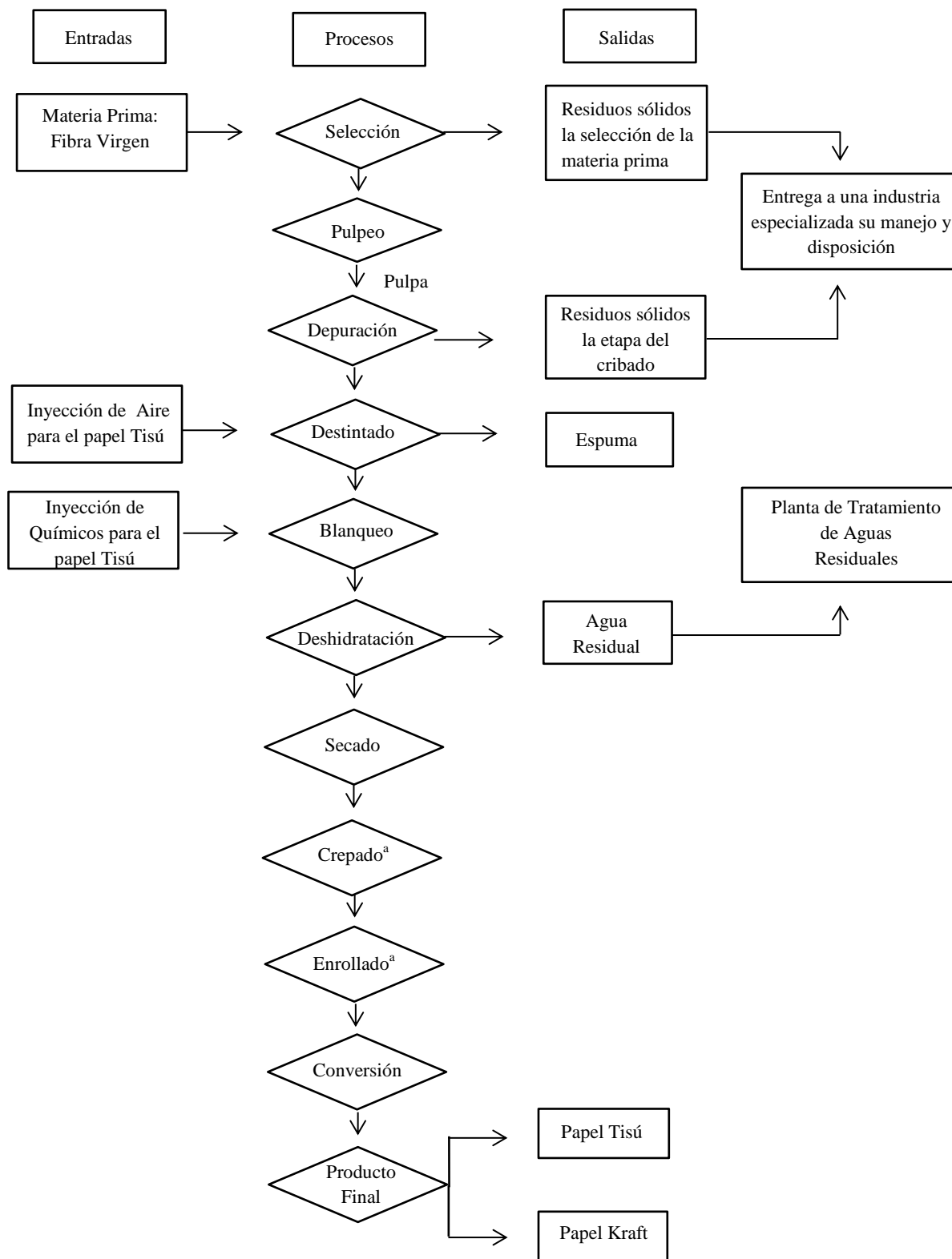
Figura 5. Diagrama del Sistema Productivo del Papel Tisú y Kraft.
