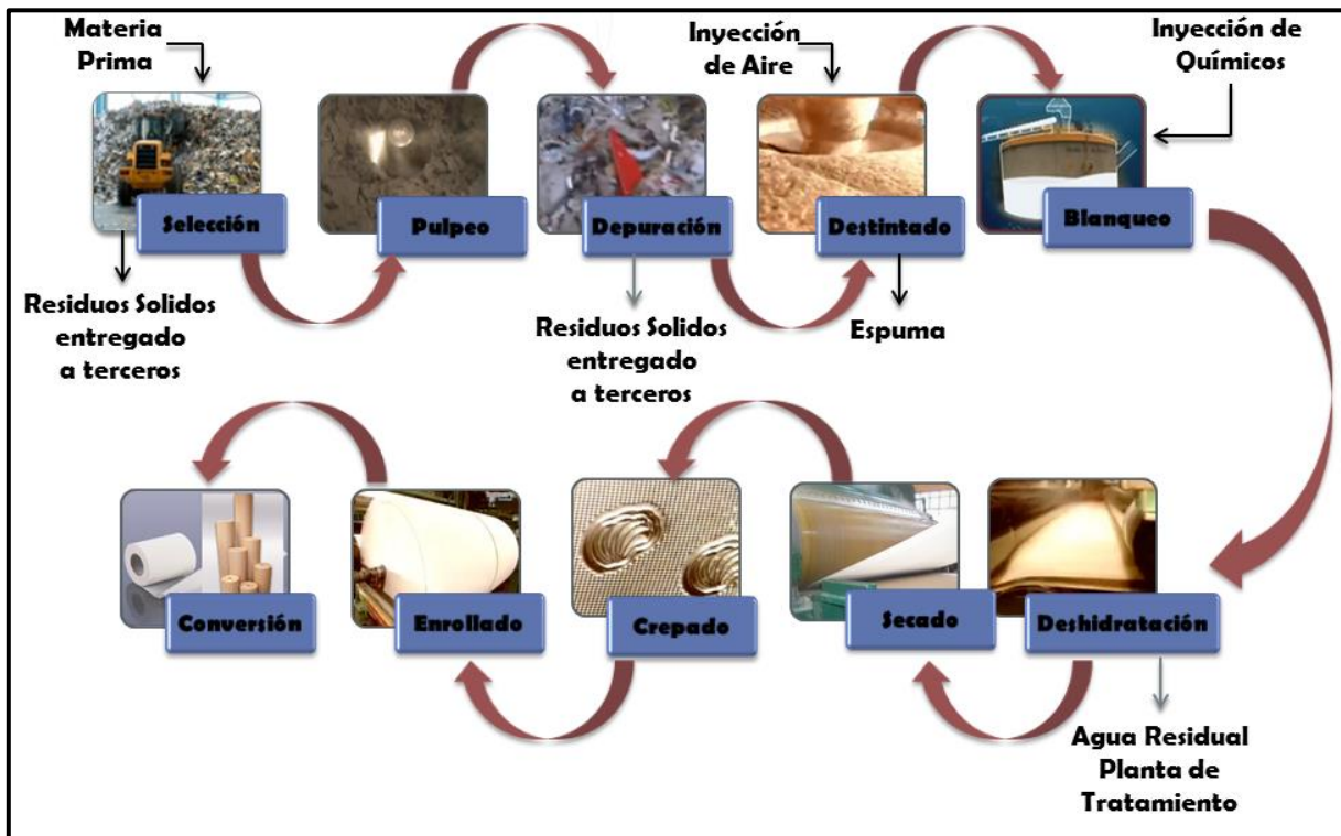
Ilustración 5. Diagrama del Sistema Productivo del Papel Tisú y Kraft
