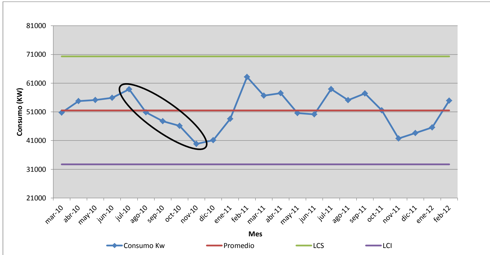
Gráfico 8. Gráfico de control sección reencauche
