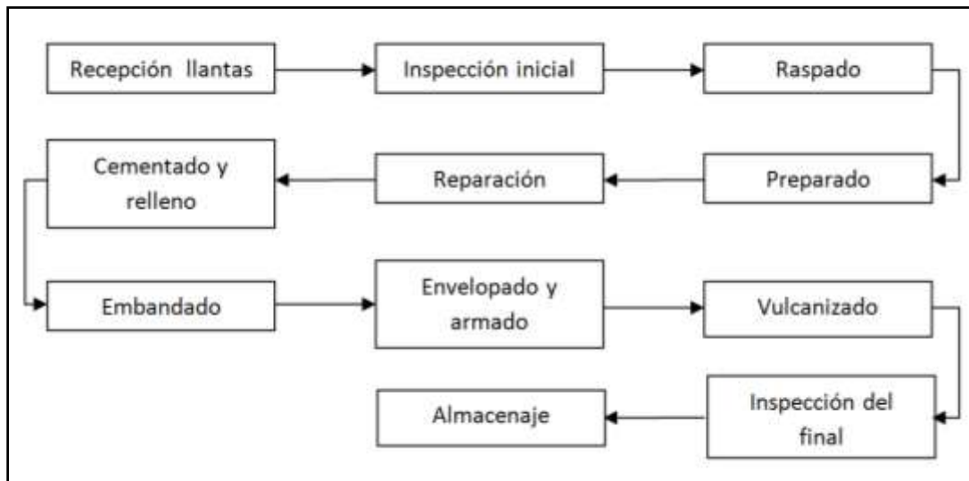
Figura 1. Diagrama de Bloques del proceso de Reencauche de Llantas
