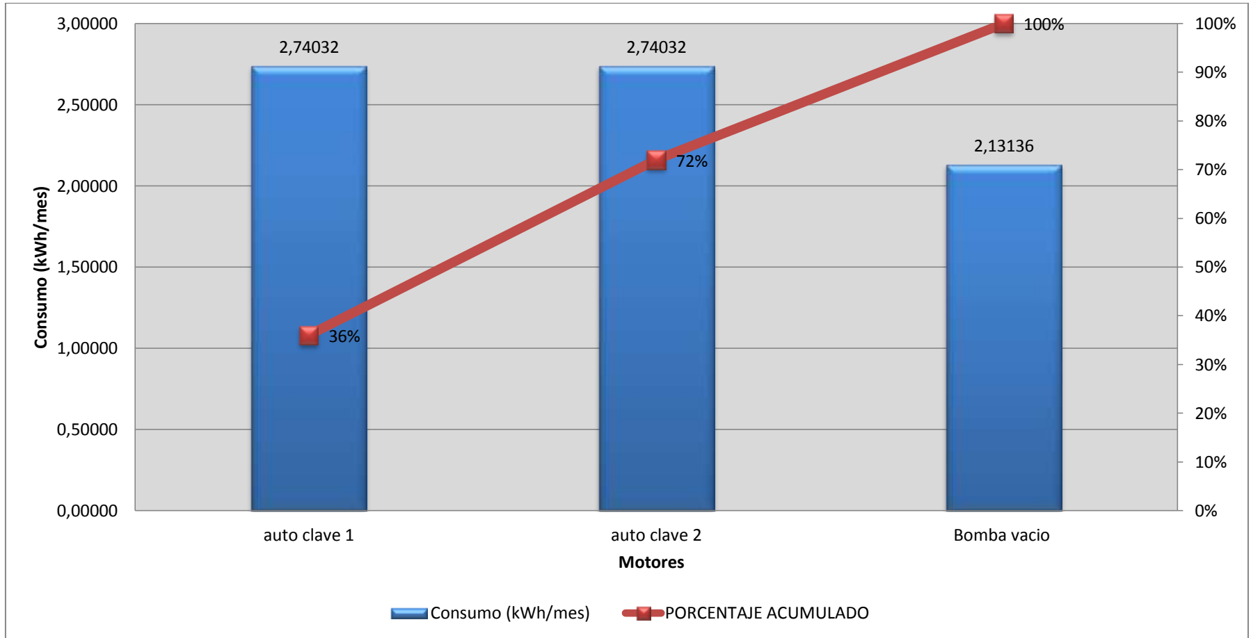
Gráfico 5. Diagrama de Pareto vulcanizado
