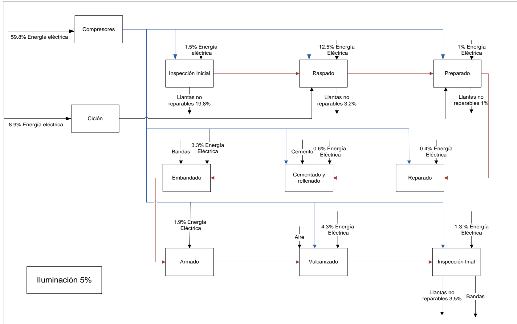
Figura 13. Diagrama energético – productivo planta
