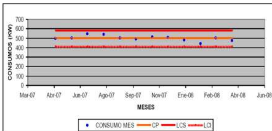
Figura 7. Gráfico de control energético.
