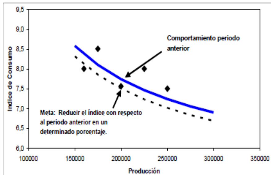
Figura 5. Índice de consumo Vs. Producción
