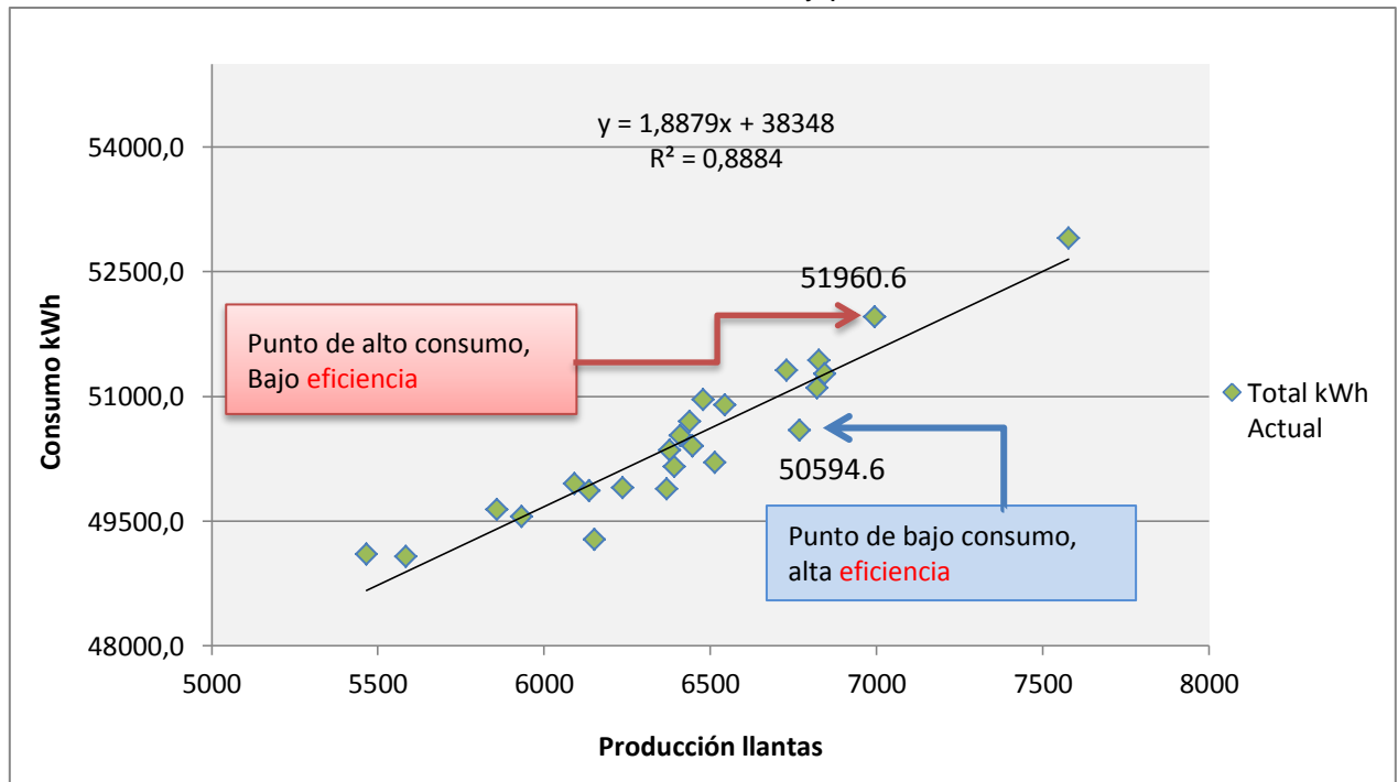
Gráfico 10. Gráfico de consumo y producción
