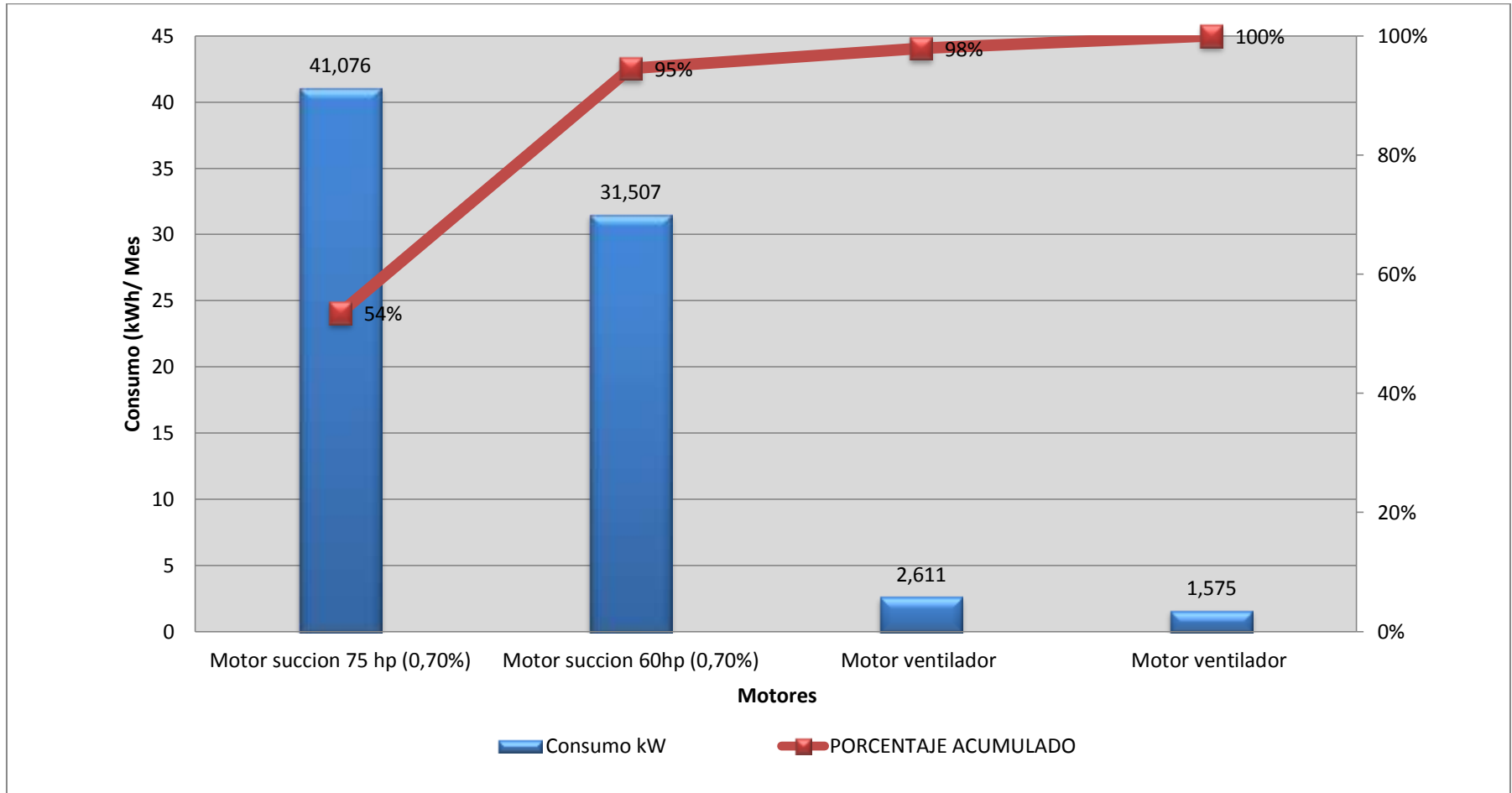
Gráfico 3. Diagrama de Pareto compresor
