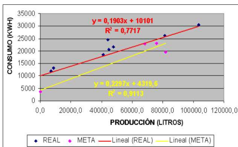
Figura 4. Gráfico de Consumo - Producción
