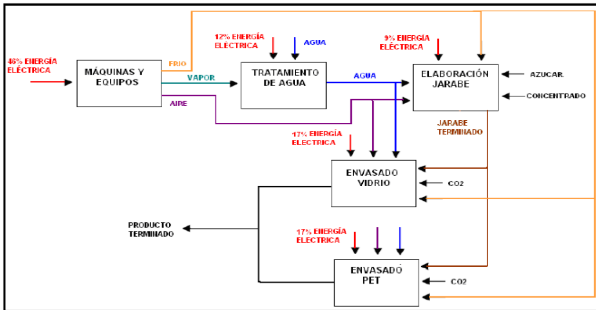
Figura 10. Diagrama Energético-Productivo.
