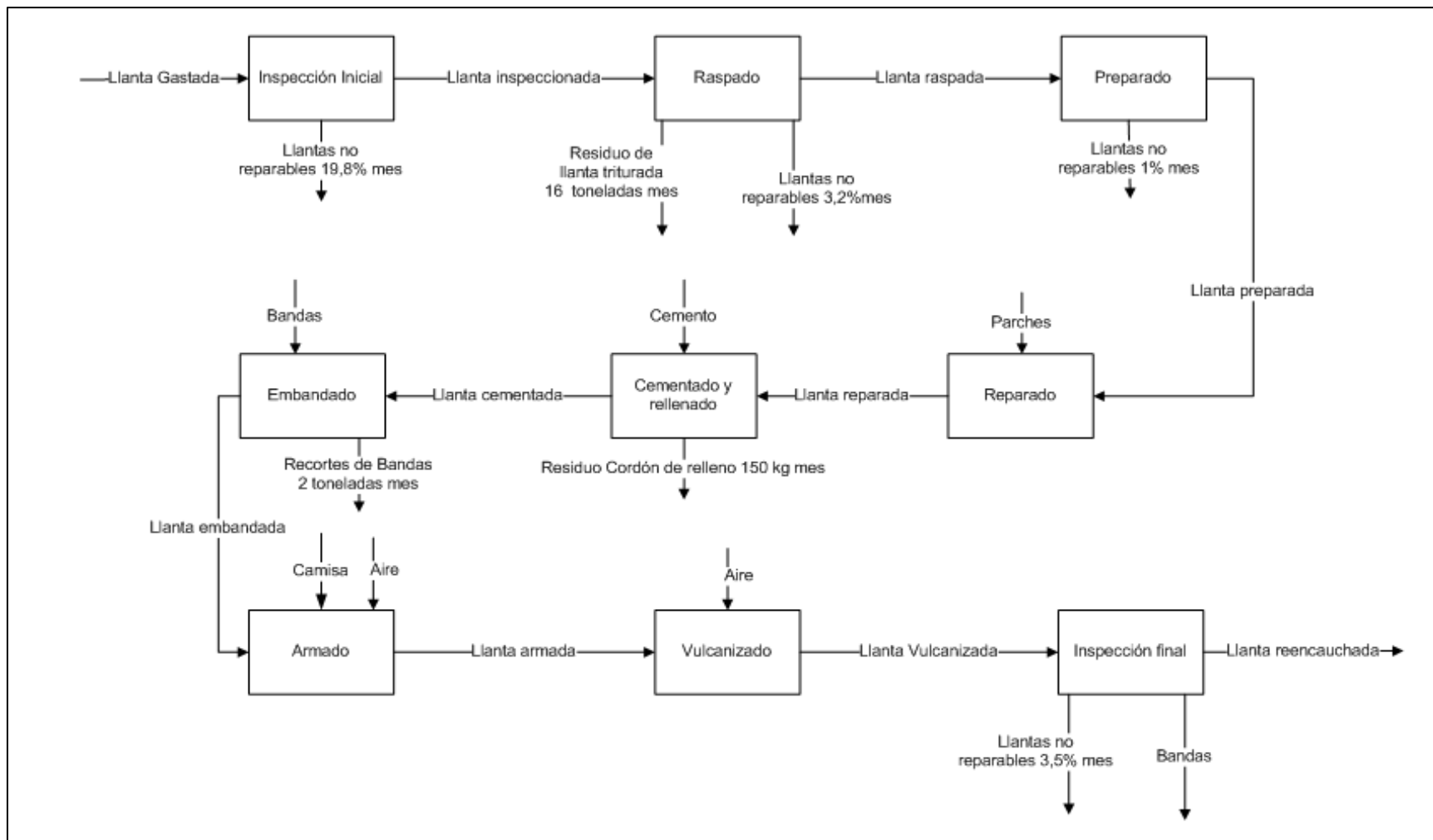
Figura 12. Diagrama de flujo proceso productivo en la sección de reencauche
