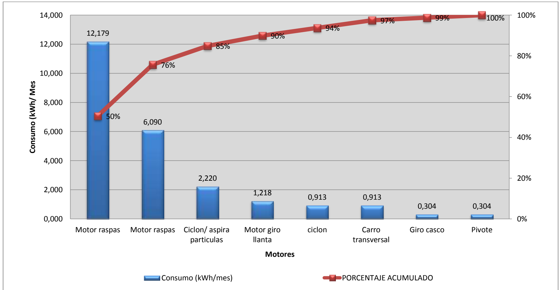
Gráfico 4. Diagrama de Pareto raspado
