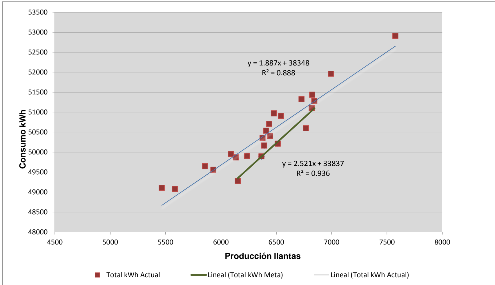
Gráfico 11. Gráfico de consumo y producción meta propuesta
