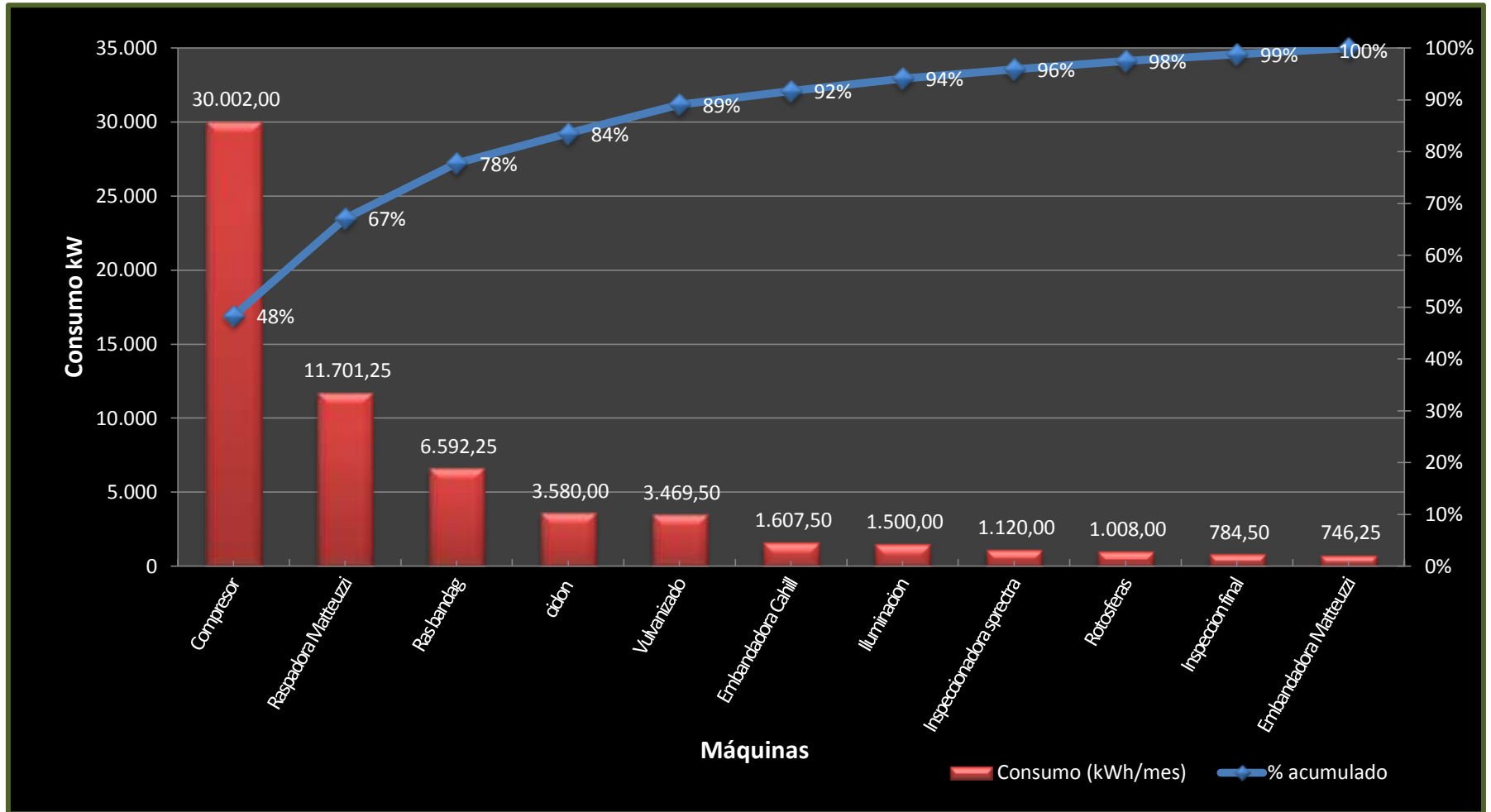
Gráfico 1. Diagrama de Pareto para la planta de reencauche teórico
