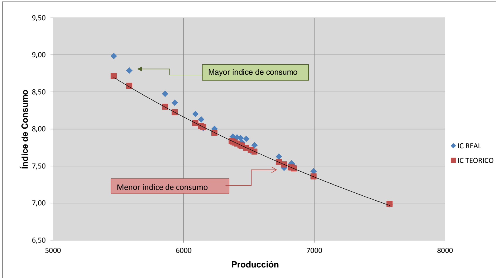
Gráfico 12. Gráfico índice de consumo y producción
