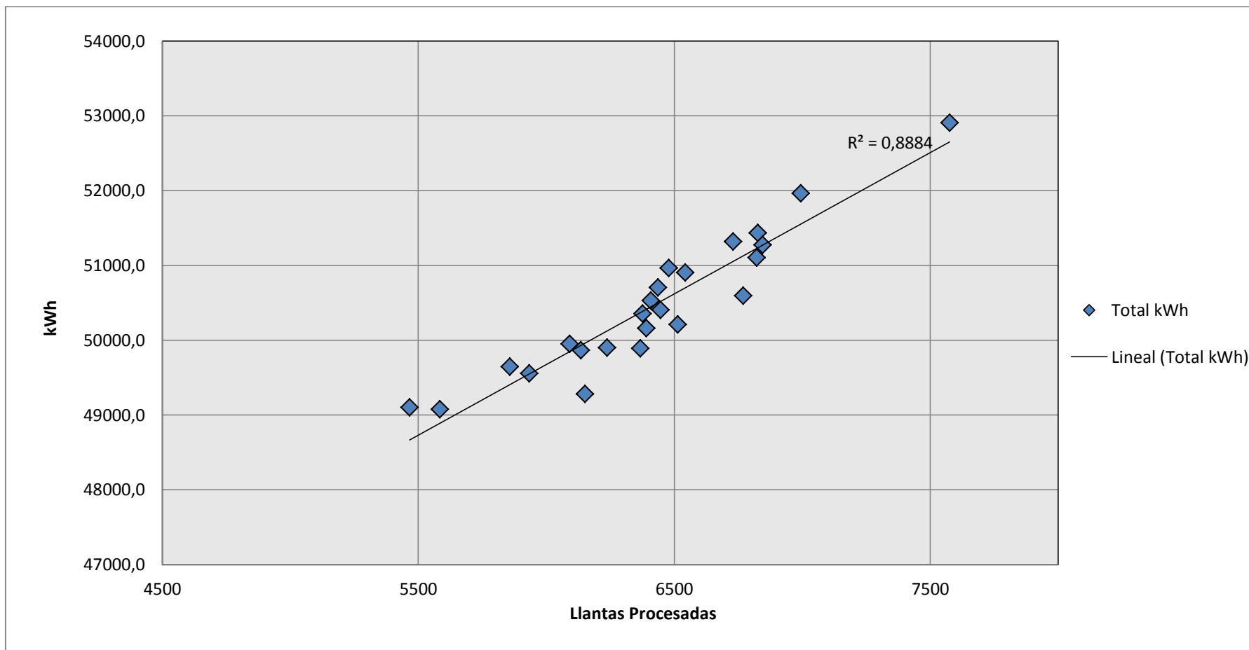
Gráfico 7. Diagrama de dispersión y correlación
