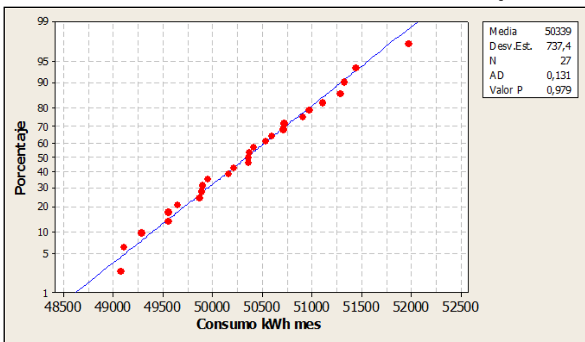
Gráfico 6. Prueba de Normalidad kWh mes – Anderson Darling
