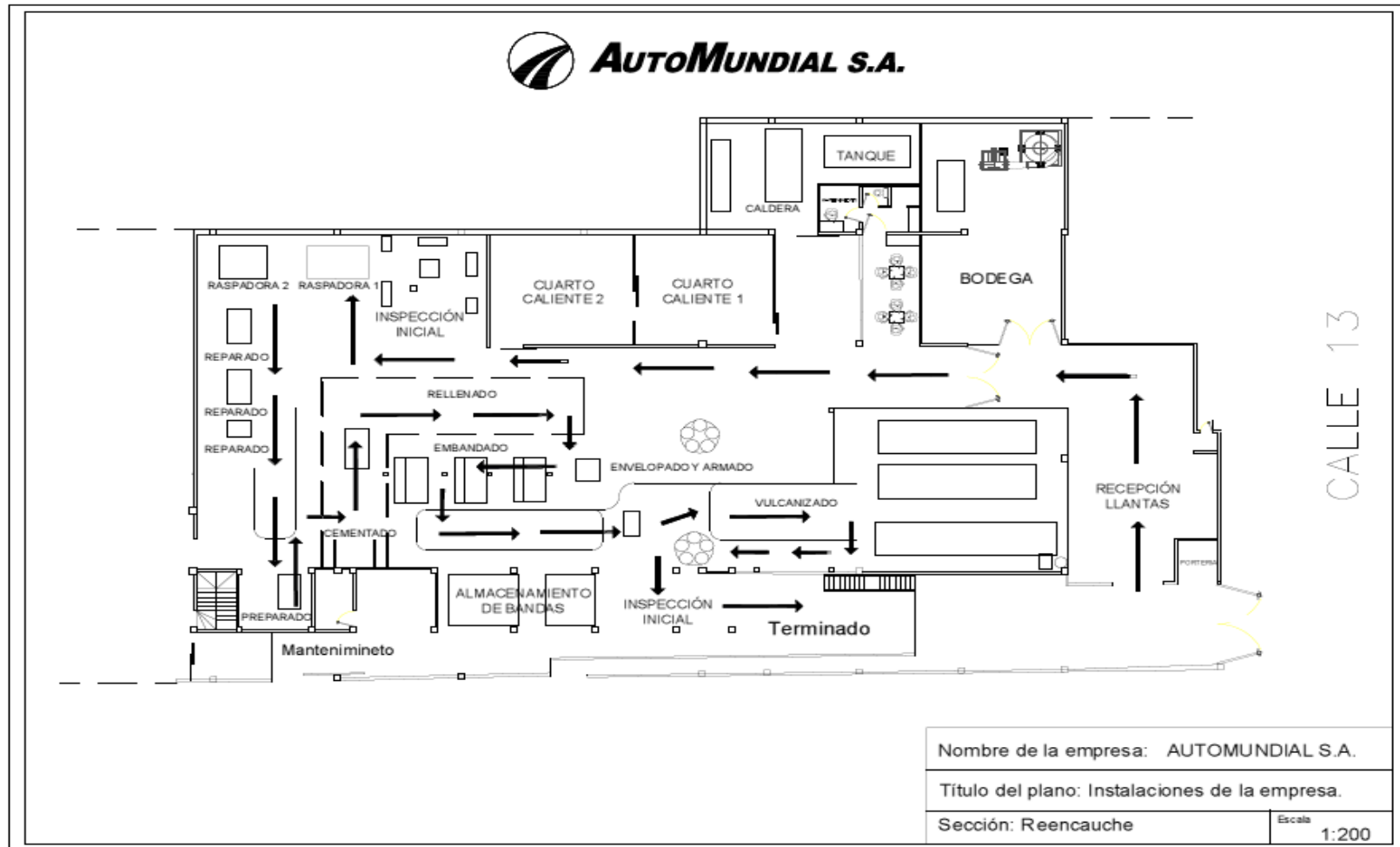
Ilustración 1. Plano Sección Reencauche
