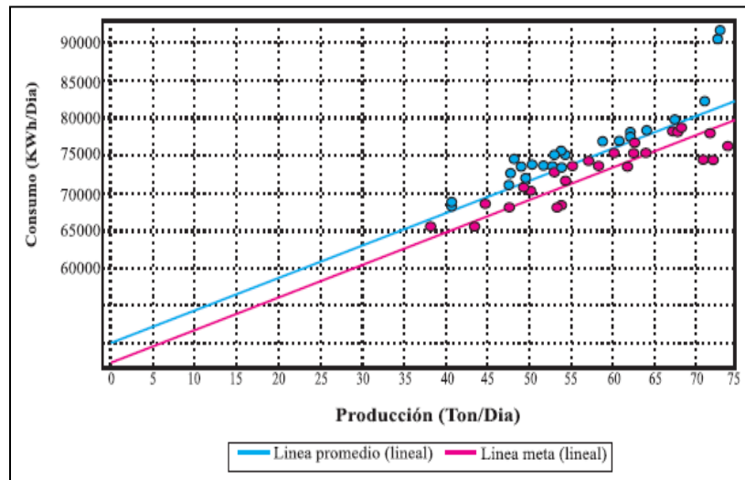
Figura 3. Diagrama de Dispersión Consumo vs Producción
