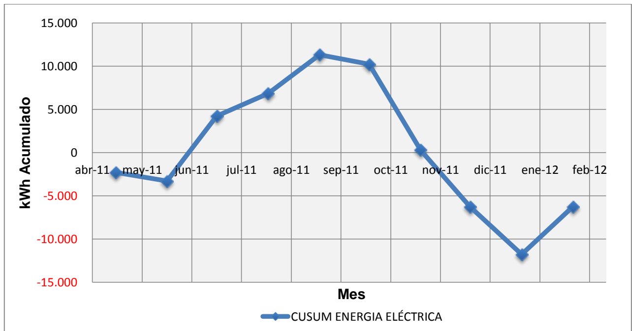
Gráfico 13. Gráfico de tendencia (CUSUM)
