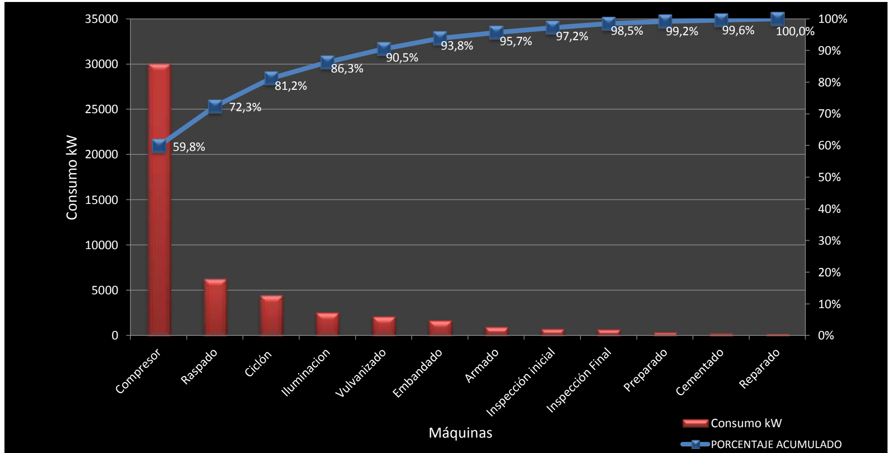
Gráfico 2. Diagrama de Pareto energía eléctrica real
