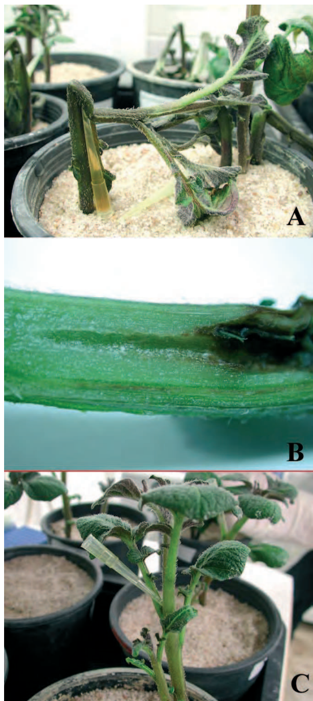
FOTO 4. Sintomas en plantas de patata inoculadas con cepas de agua de Dickeya spp.:
