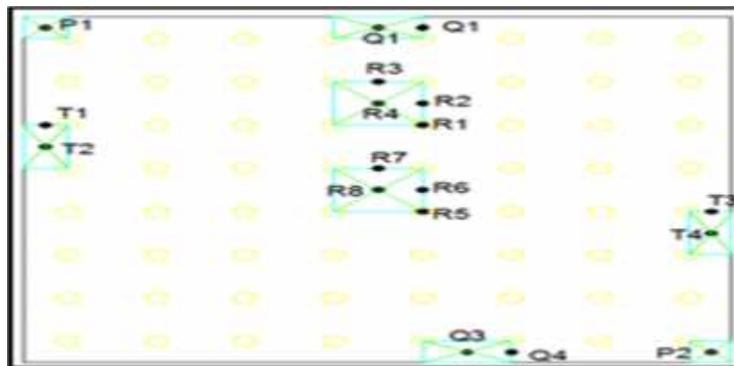
Figura9. Puntos de medición de iluminancia en la cuadrícula de un local con luminarias espaciadas simétricamente en dos o más filas
