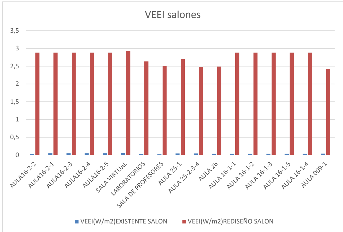
Figura77. Grafica estadística de la VEEI en los espacios representados en las imágenes anteriores
