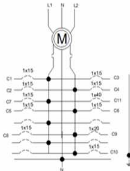
Figura15. Diagrama unifilar tablero 1
