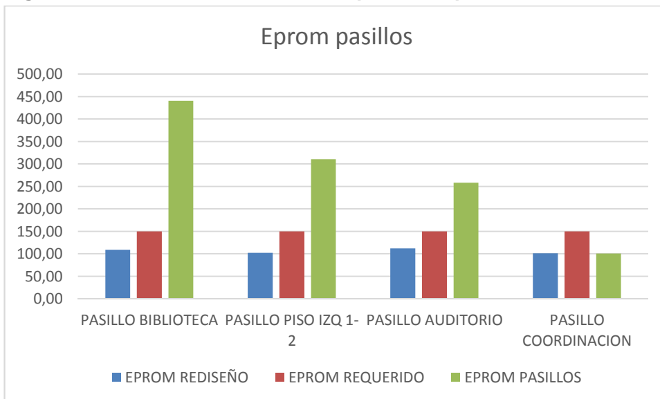
Figura54.Resultados de iluminancia promedio pasillos
