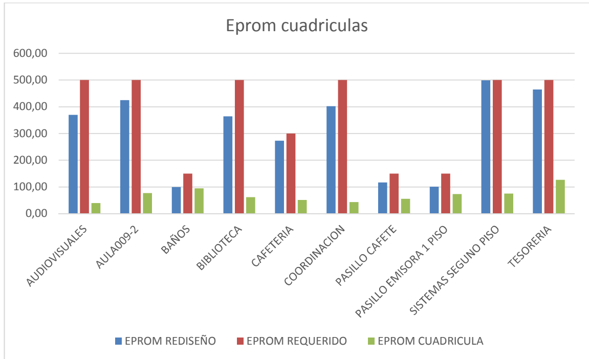
Figura66 Resultados de iluminancia promedio en los espacios representados en las imágenes anteriores
