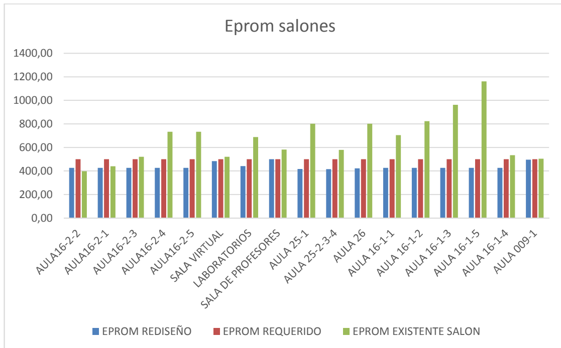
Figura76. Resultados de iluminancia promedio en los espacios representados en las imágenes anteriores
