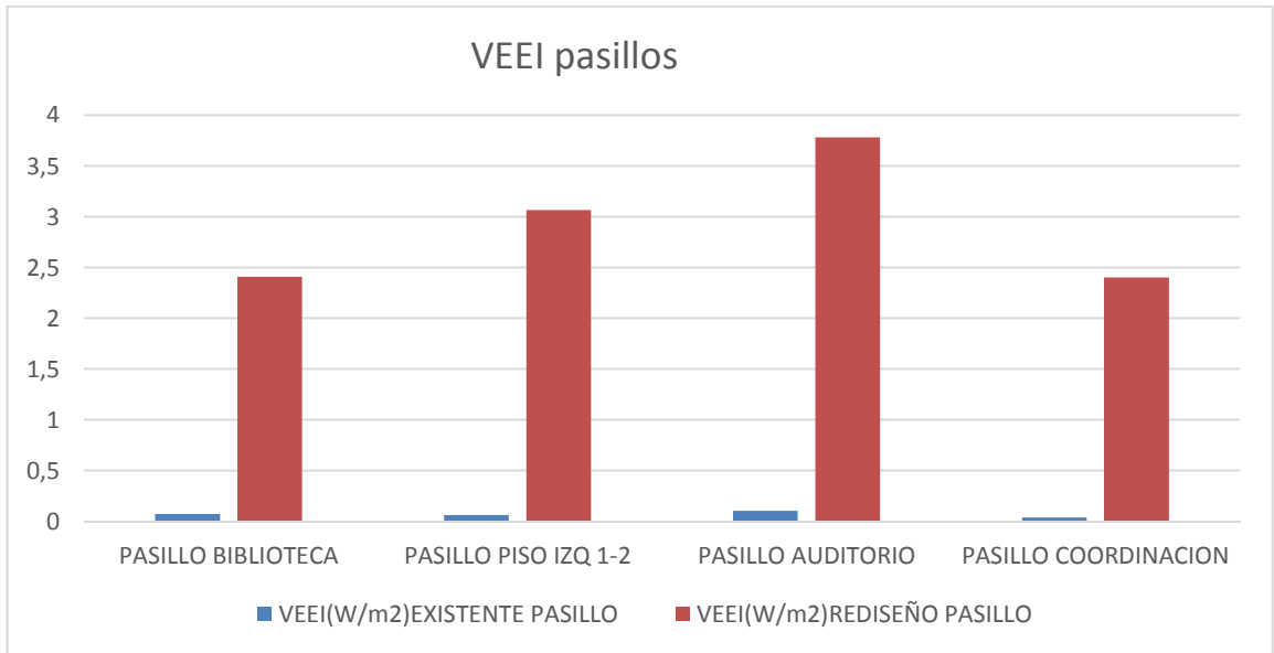
Figura55. Grafica estadística de la VEEI pasillos
