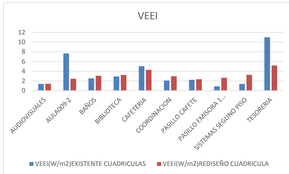
Figura67. Grafica estadística de la VEEI en los espacios representados en las imágenes anteriores
