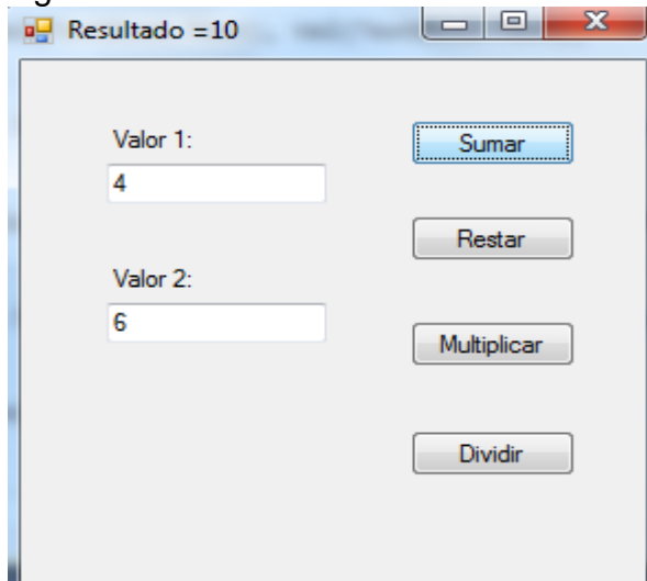
Figura 5. Calculadora sumando
