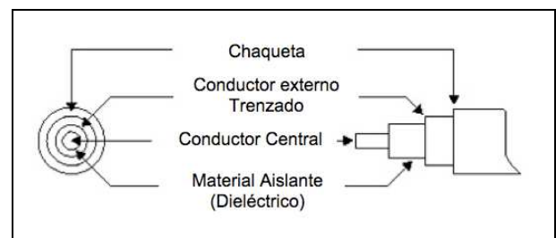
Figura 3. Construcción del cable coaxial
