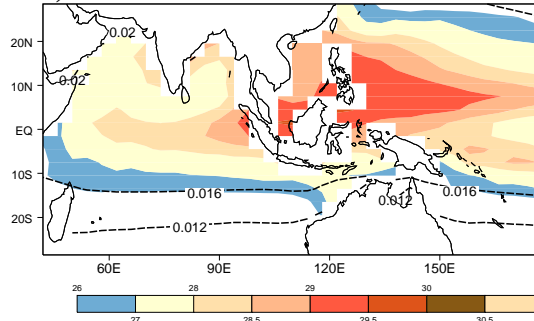
p) MIROC3.2 (hires)
