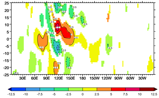
n) GISS-AOM
