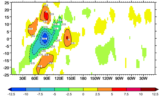
n) GISS-AOM
