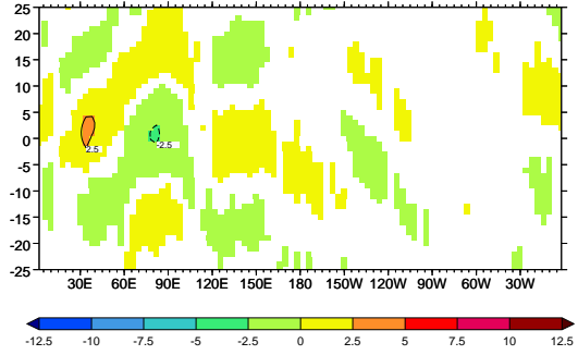
p) MIROC3.2 (hires)
