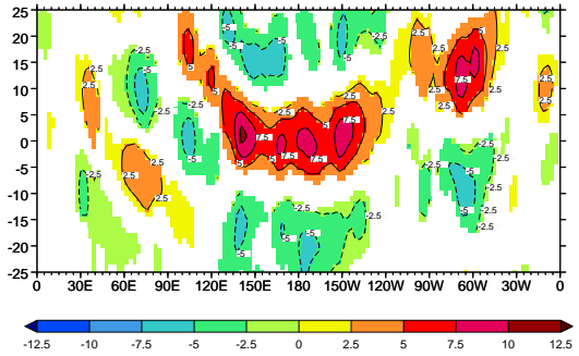
j) ECHO-G (MIUB)
