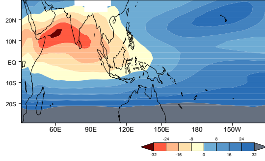
q) MIROC3.2 (medres)
