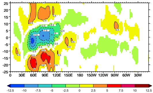
r) MRI-CGCM2.3.2
