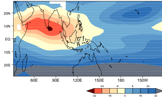
n) GISS-AOM
