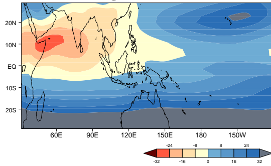
m) GFDL-CM2.1
