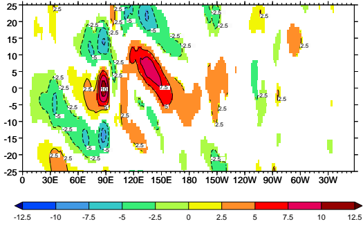
i) ECHO-G
