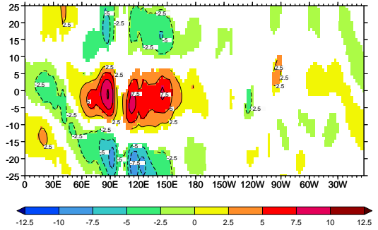
r) MRI-CGCM2.3.2
