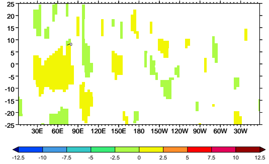
p) MIROC3.2 (hires)
