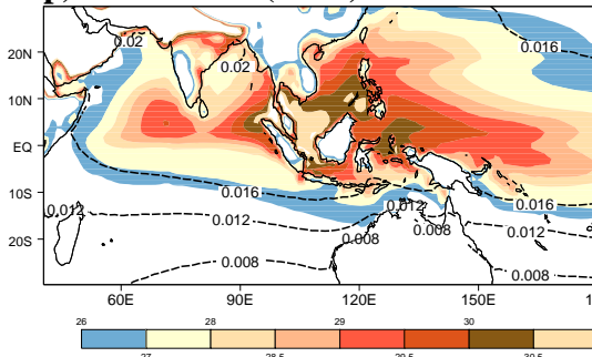
r) MRI-CGCM2.3.2
