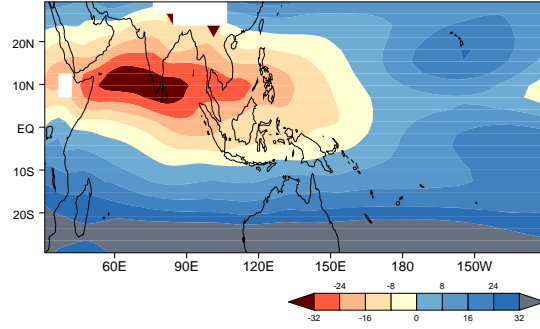
r) MRI-CGCM2.3.2
