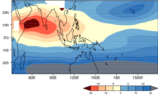
o) IPSL-CM4
