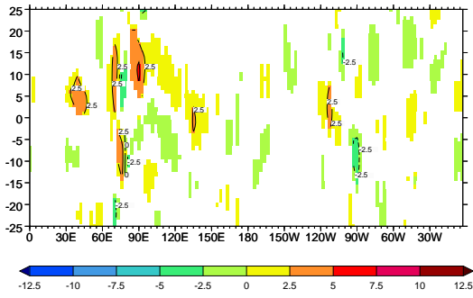
m) GFDL-CM2.1
