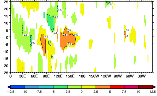
f) CSIRO MK3.0
