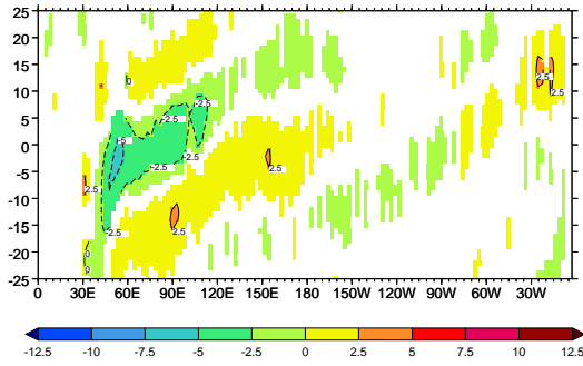
m) GFDL-CM2.1
