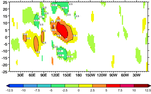
o) IPSL-CM4
