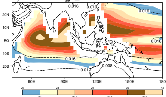
m) GFDL-CM2.1
