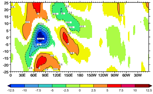
h) ECHAM4/OPYC
