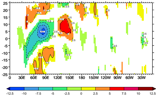
g) ECHAM5/MPI-OM
