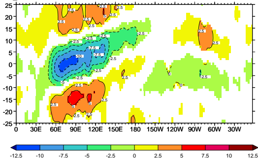
q) MIROC3.2 (medres)
