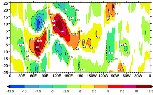
c) CGCM3.1 (T47)
