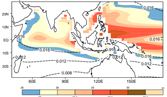
o) IPSL-CM4
