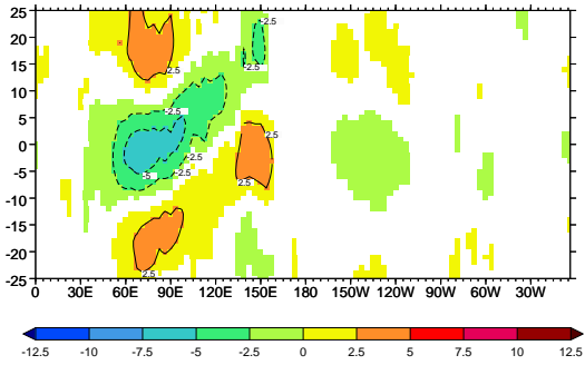
e) CNRM-CM3
