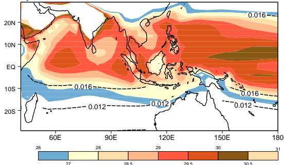
q) MIROC3.2 (medres)
