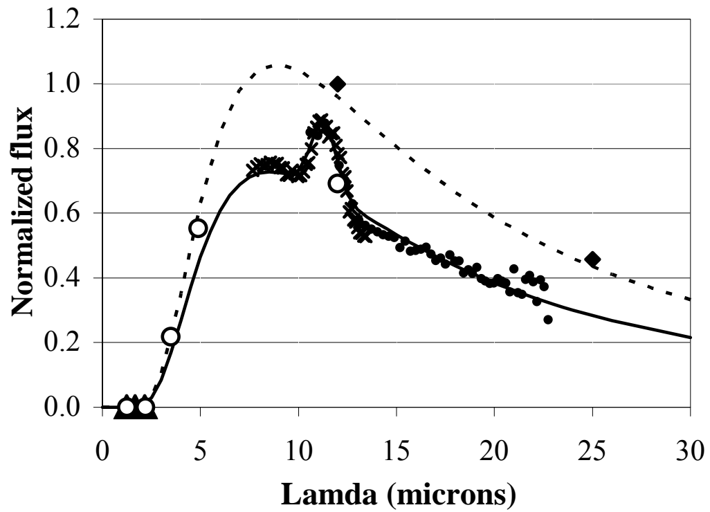
Fig. 1: IRAS 17446-4048
