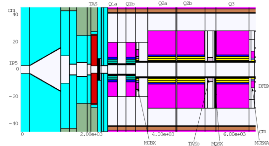
Figure 5. SYM-1 longitudinal MARS model.
