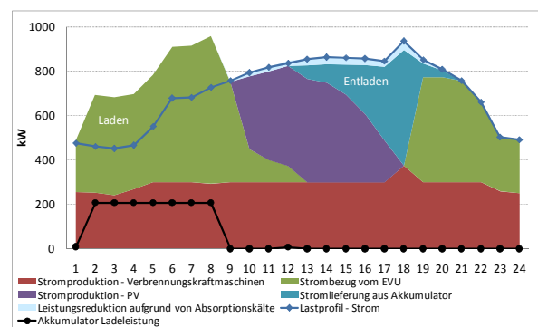
Abbildung 3: Deckung der Pflegeheim Stromlast an einem Juli Wochentag. Quelle: 2) und 3)
