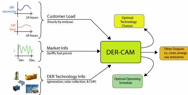
Abbildung 1: DER-CAM Strukturplan. Quelle: 2)
