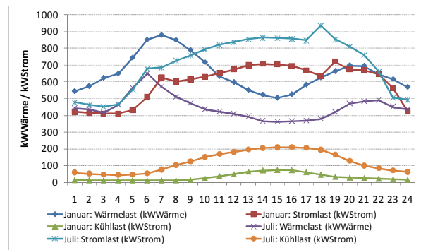
Abbildung 2: Strom- und Wärmelasten an Juli und Januar Wochentagen. Quelle: 2) und 3)
