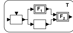
b). Workflow Template T(F_1, F_2)
