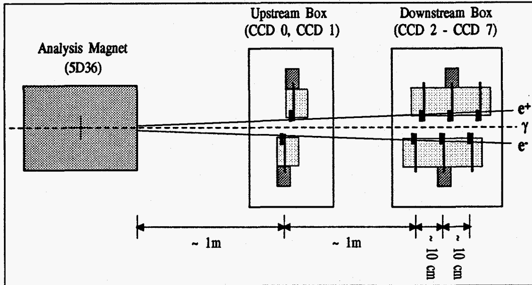
Fig. 9. The CCD pair spectrometer.
