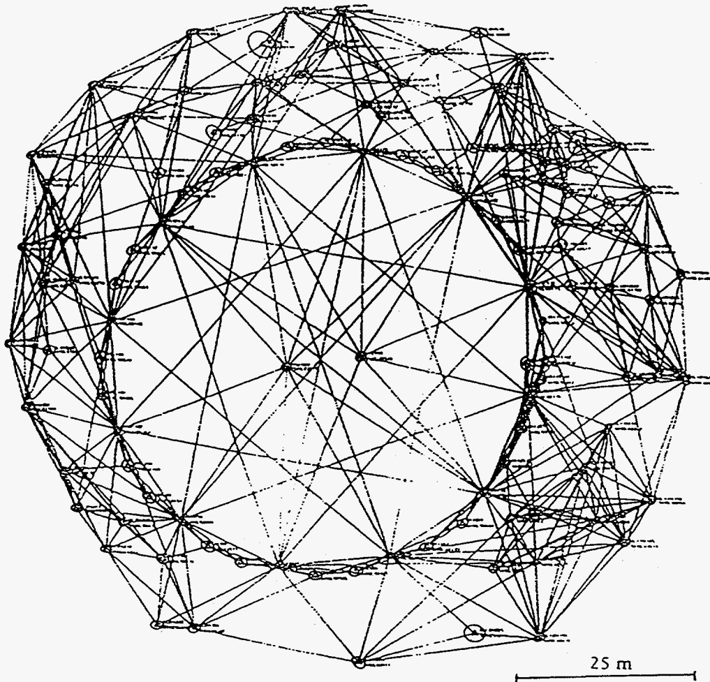
Figure 4 The ALS Monument Network 1995
