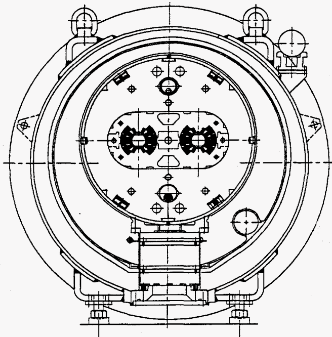
Fig. 2 LHC dipole
