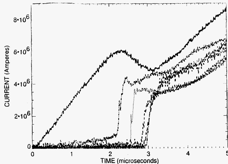
Figure 9. Magnetic Probe Signals in the Power Flow Channel. (— 01, - · - · 02, · · · · 04, - - - 06, - - 08, - · · · 010).
