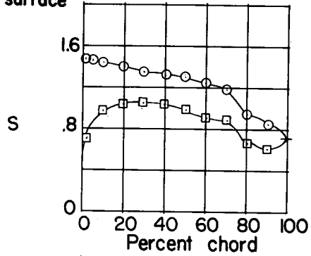
(d) \alpha_1 = 10.0^\circ ; \theta = 12.4^\circ
