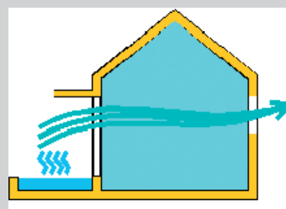
Fig. 59 – Arrefecimento Evaporativo
