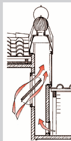
Fig. 53 – Chaminé Solar
