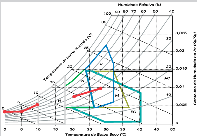
Figura 28 – Carta Bioclimática para a cidade de Bragança (I 3 V 2 )
