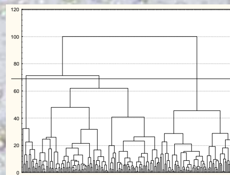
Figura 1 - Dendograma
