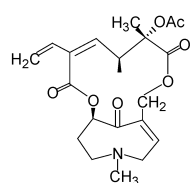
Clivorine
