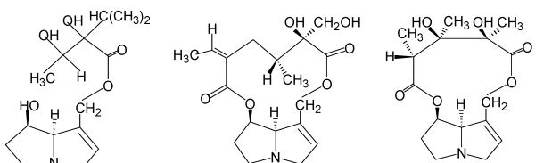
Lycopamine
