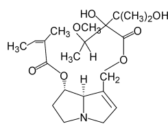
Lasiocarpine
