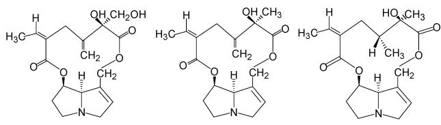
Riddelliine
