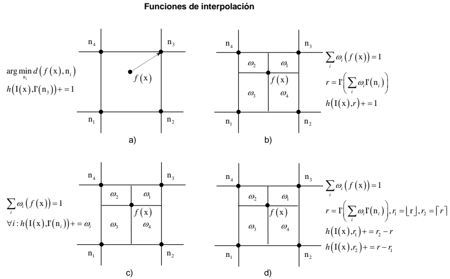
Figura 2.10: Funciones de interpolación: (a) “vecino más próximo” (b) bilineal, (c) volumen parcial y (c) interpolación parcial.
