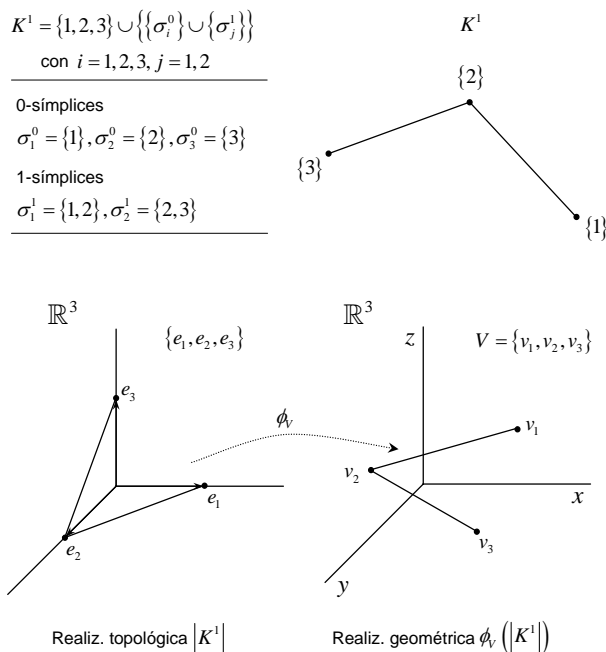
Figura C.5: Realización topológica y geométrica de un complejo simplicial.
