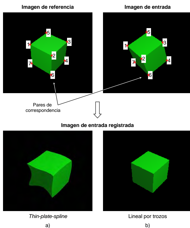
Figura 4.1: Registro de un par de imágenes de una escena poliédrica mediante una transformación: (a) thin-plate-spline y (b) lineal por trozos. Obsérvese la precisión de la transformación lineal por trozos, mientras que la thin-plate-spline produce una imagen registrada con importantes distorsiones.
