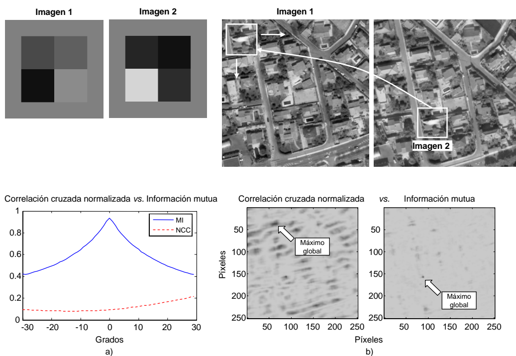
Figura 2.4: Experimentos que ilustran la idoneidad de la MI frente a la NCC como medida de consistencia. (a) Un patrón sintético es rotado (desde -30^\circ hasta +30^\circ ) sobre otro con la misma estructura (esto es, un cuadro de igual tamaño) pero con distintos niveles de gris; y (b) un pequeño trozo de una imagen de satélite QuickBird es desplazado sobre otra imagen de la misma escena adquirida en otra fecha. Obsérvese como, a diferencia de la MI, la NCC falla en ambos experimentos, esto es, no detecta un máximo global en (a) y proporciona un máximo global erróneo en (b).
