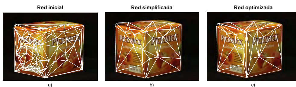
Figura 5.14: Red triangular optimizada con el método propuesto: (a) red inicial, (b) red simplificada (sólo acciones de eliminación) y (c) red optimizada (todas las acciones). Obsérvese como, dada la disposiciones de las correspondencias, no ha sido necesaria la inclusión de nuevos vértices.
