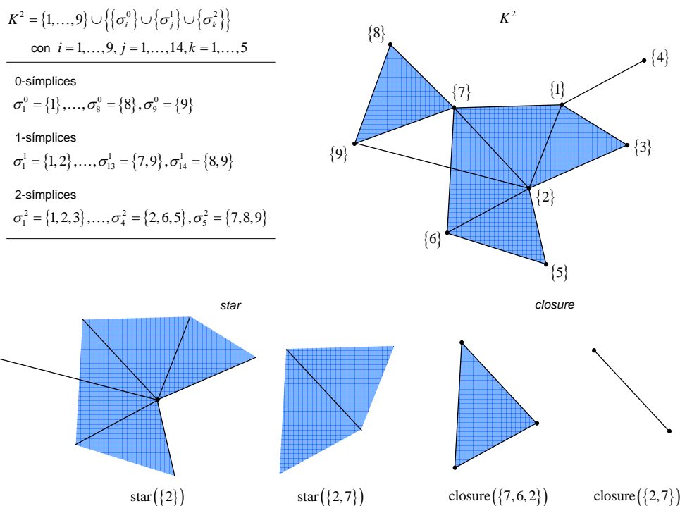
Figura C.3: Ilustración de un complejo simplicial abstracto de dimensión 2 y algunos de sus subconjuntos: estrella, cierre.
