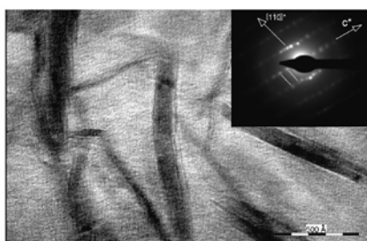
fig.4. Imagen de alta resolución mostrando el espaciado de las partículas de tobelita de la reacción 1. Arriba a la derecha SAED que muestra un paquete de politipo 1M.
