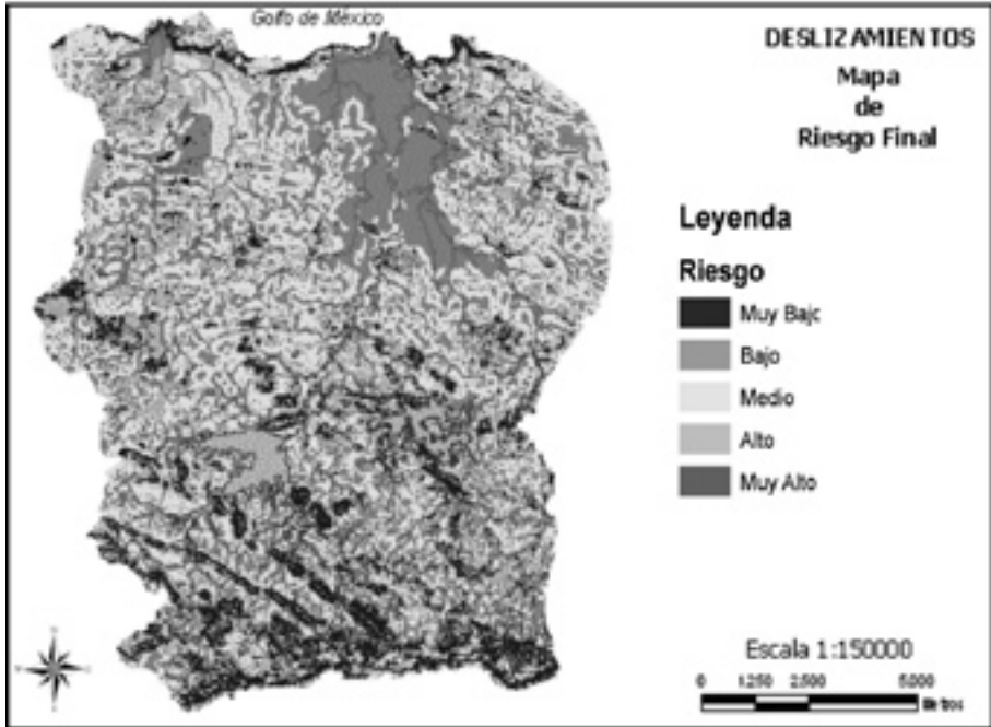
FIGURA 9 RIESGOS DE DESLIZAMIENTOS Y FENÓMENOS DE LADERA
