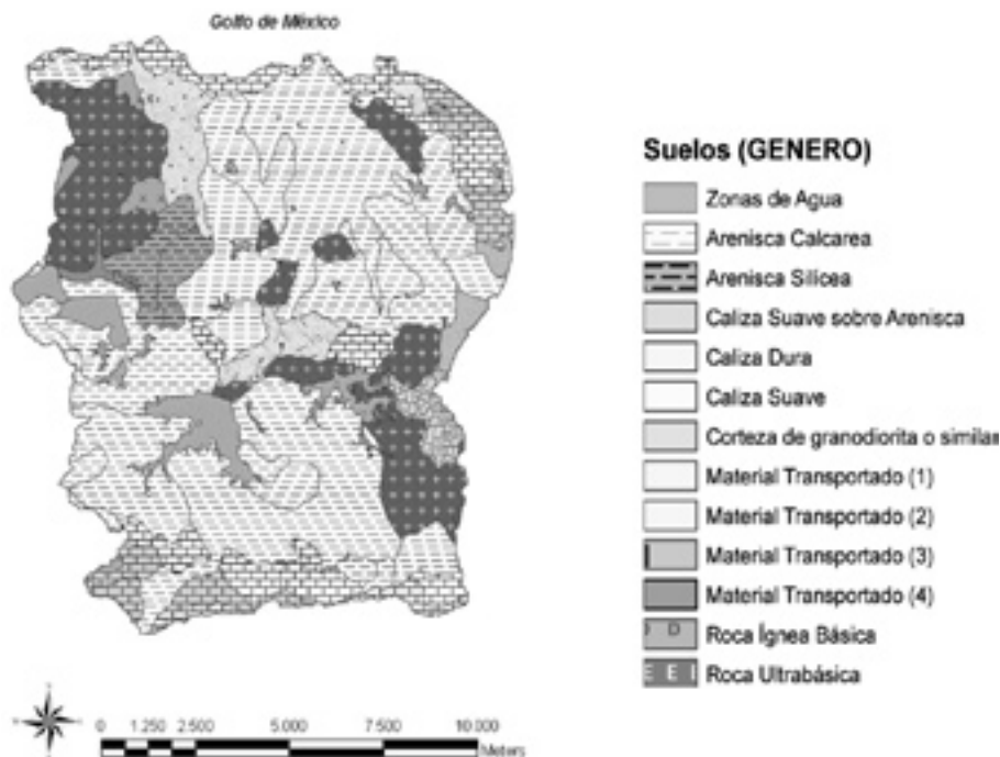
FIGURA 2 SUELOS SEGÚN SU LITOLOGÍA
