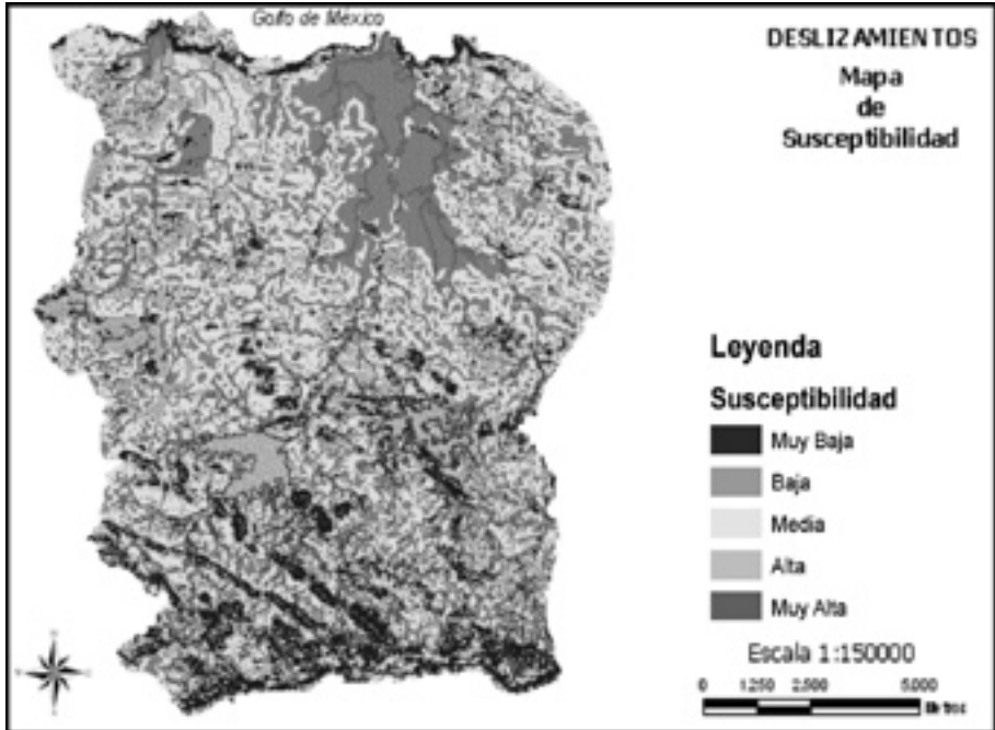
FIGURA 7 SUSCEPTIBILIDAD A DESLIZAMIENTOS
