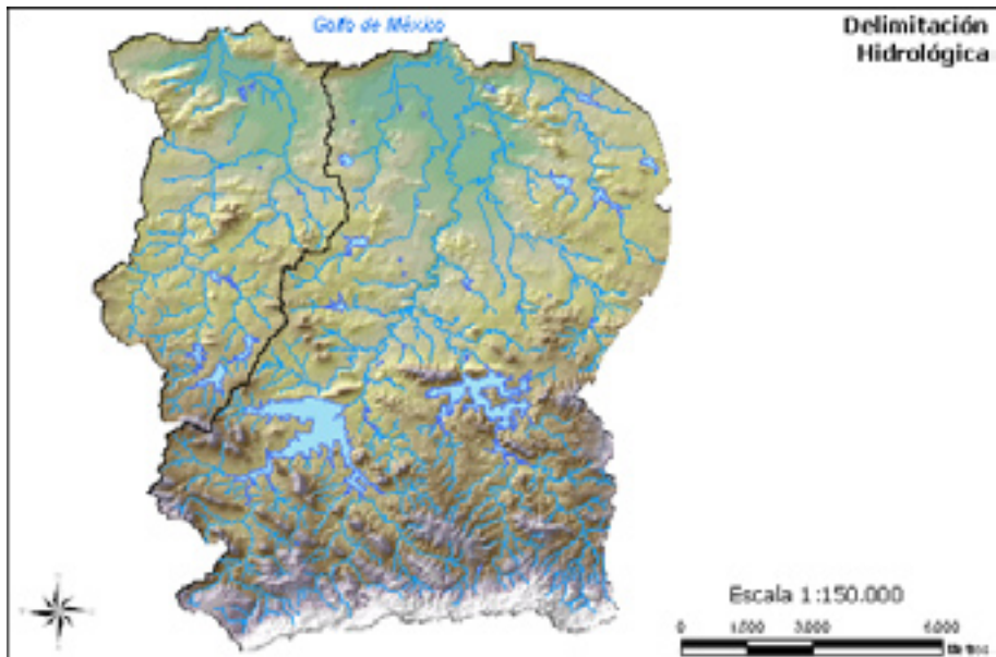
FIGURA 4 CUENCAS HIDROLÓGICAS
