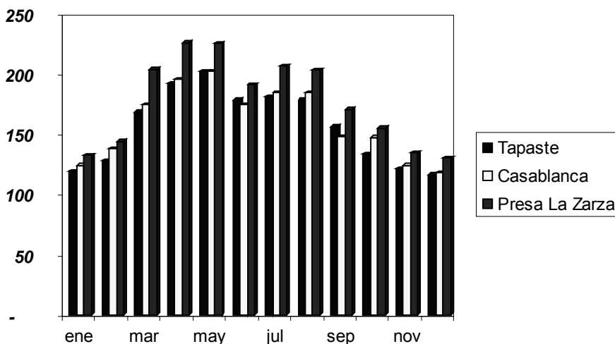
FIGURA 14 EVAPORACIÓN INTRA-ANUAL DESDE LA SUPERFICIE LIBRE DEL AGUA EN LAS ESTACIONES CASABLANCA, PRESA LA ZARZA Y TAPASTE. PERÍODO 1970-1995
