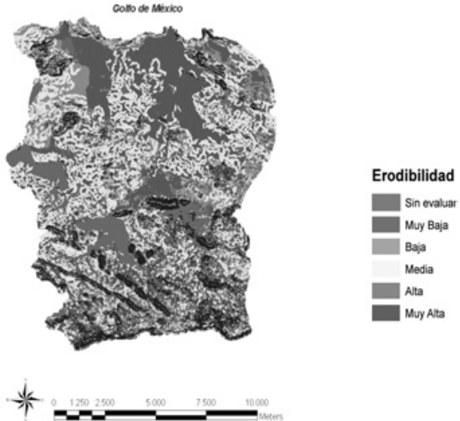
FIGURA 6 ERODIBILIDAD DE LOS SUELOS
