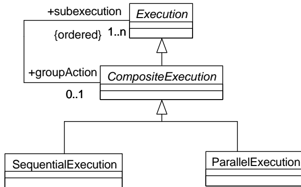
Figura 2.10: Paquete de conceptos de instancias de las acciones compuestas (compositeactions.instance.concepts).
