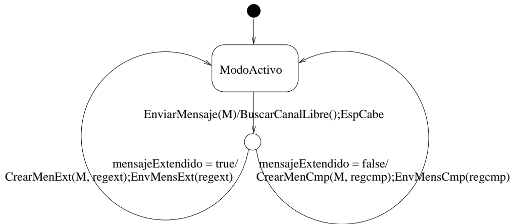
Figura 4.8: Máquinas de estados del objeto DComboSa1.
