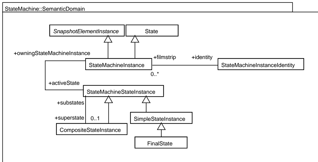
Figura 3.8: Dominio semántico de las máquinas de estados con estados compuestos.
