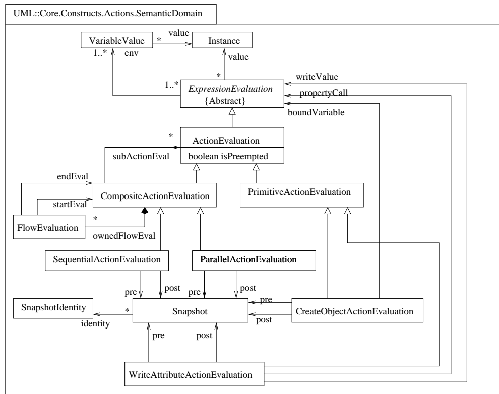
Figura 2.16: Dominio semántico del paquete Actions donde los estados pre- y posteriores de todas las acciones son de la clase Snapshot
