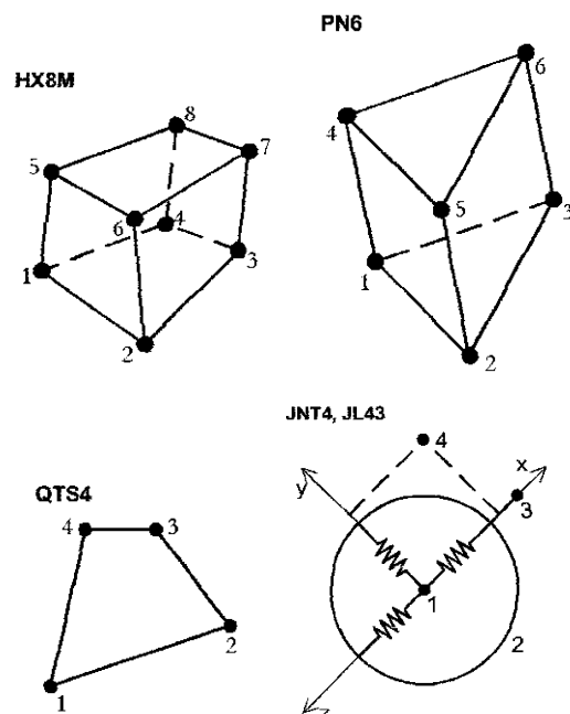
Fig. 7 - Elementos finitos.
