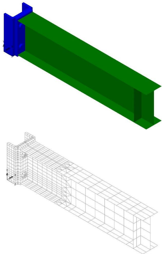
Fig. 5 - Modelo numérico.
