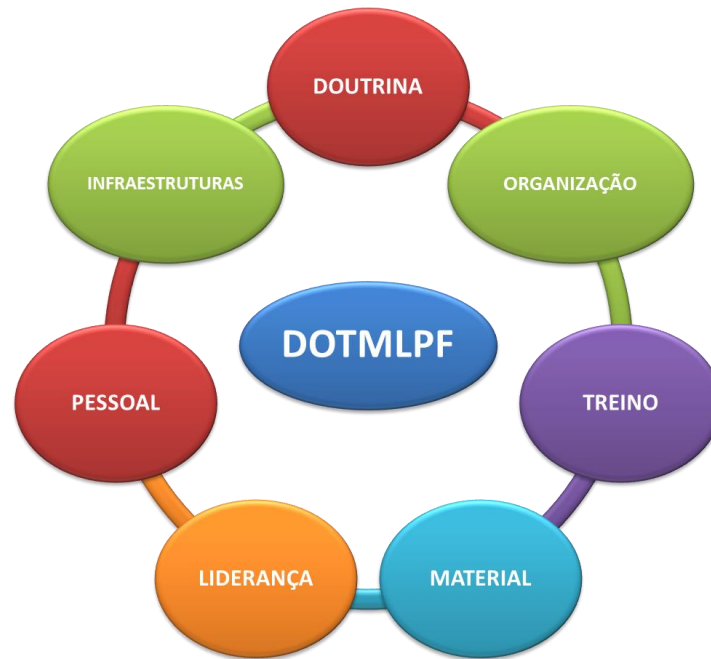
Figura nº 6 – Modelo DOTMLPF
