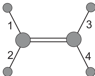
Fig. 7. Ethene
