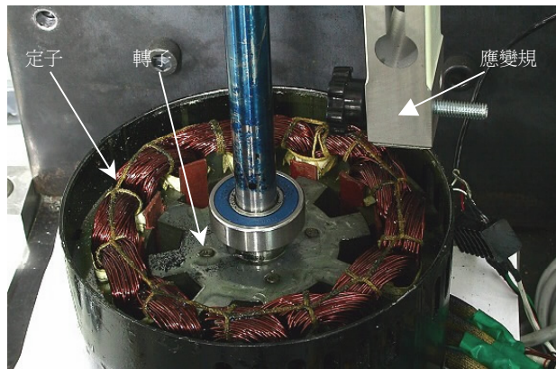
圖 7、馬達內部圖
