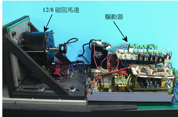
圖 6、磁阻馬達外觀與自驅動器
