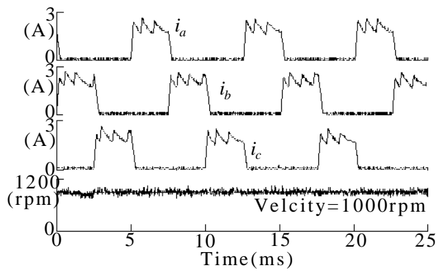
圖 8、1000 rpm，1 Nm，三相電流
