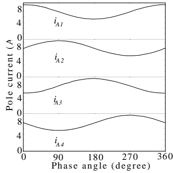
圖 3、 \theta_f 從 0 度~360 度時 A 相之四個極的激磁電流
