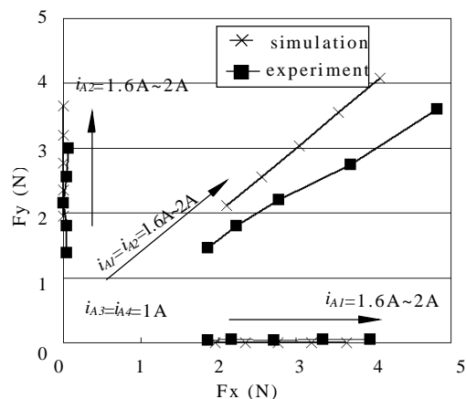
圖 9、Ansoft 計算與實測之徑向力比較
