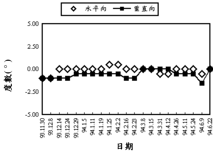
圖 34 5 號監測點之傾度盤量測值
