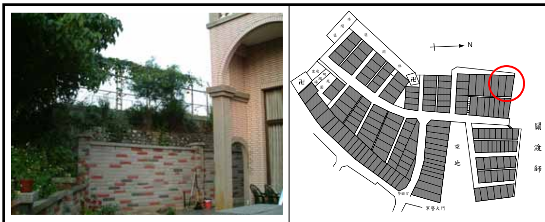
圖 6 現場照片及概要說明：營區鄰近社區之擋土牆，就其外觀尚屬穩定安全，但其下方為陡峭之邊坡，故其排水、水壓狀況和潛勢仍須監控。
