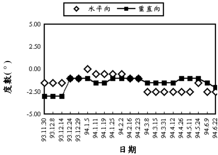
圖 31 2 號監測點之傾度盤量測值
