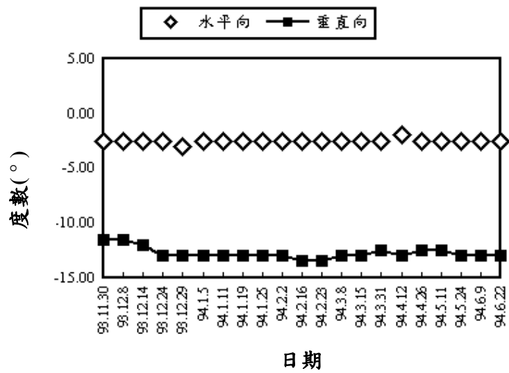
圖 35 6 號監測點之傾度盤量測值
