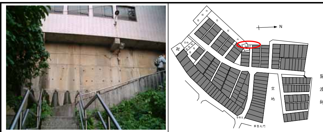
圖 7 現場照片及概要說明：東北側之社區下方擋土牆之排水孔，須定期檢視其排水情況。
