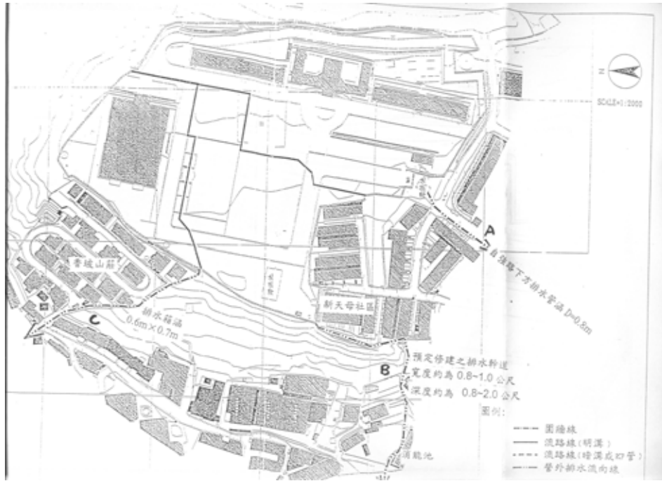
圖 4 第一年期社區外圍排水系統圖
