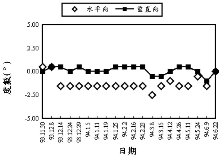
圖 32 3 號監測點之傾度盤量測值
