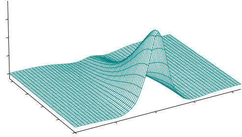
圖一、邊緣荷重下兩相鄰版之撓度示意圖
