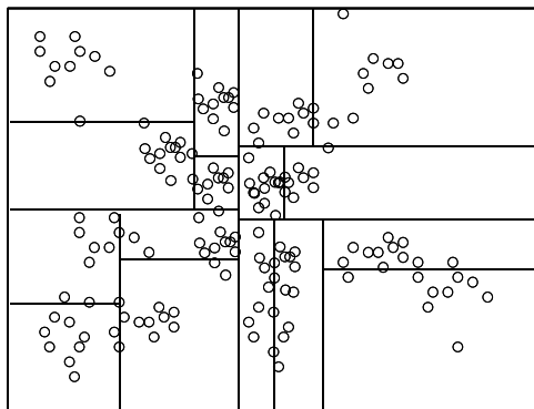
圖三、LOESS 小區域分割示意圖
