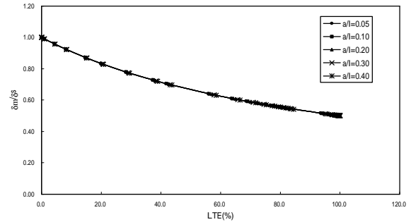
圖二、荷重傳遞修正因子關係圖
